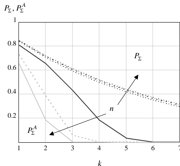
Рисунку 5 – Сімейства залежностей імовірності правильної роботи пристрою та імовірності успішної атаки на криптопристрій
