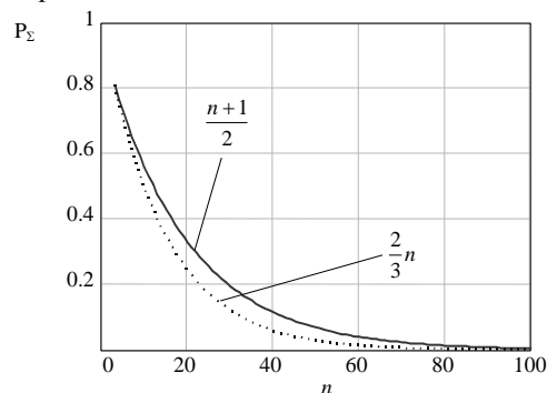
Рисунок 3 – Імовірність успішного виконання атаки апаратних помилок для криптопристроїв, що використовують різні мажоритарні функції
