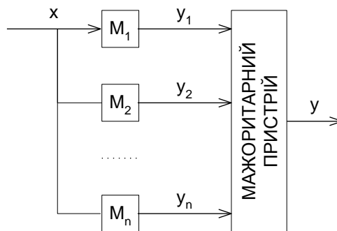
Рисуюнок 1 - Узагальнена архітектура традиційного резервування з однотипними модулями
