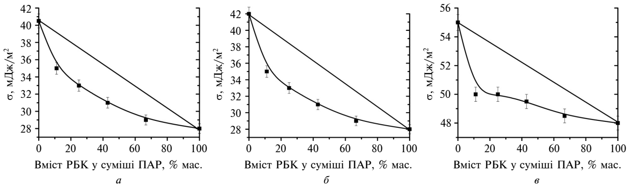
Рис. 2. Залежність поверхневого натягу водних розчинів сумішей Tween-80 і РБК від вмісту РБК на ділянках концентрацій: а – більший за ККМ (1,25–10 %), б – близький до ККМ (0,625 %), в – менший за ККМ (0,004 %), від загальної кількості ПАР у розчинах
