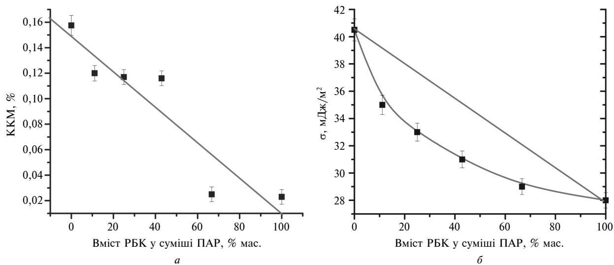
Рис. 3. Залежності ККМ (а) та поверхневого натягу (б) від вмісту РБК (%) у водних розчинах сумішей ПАР (загальна концентрація ПАР 10 г/л)
