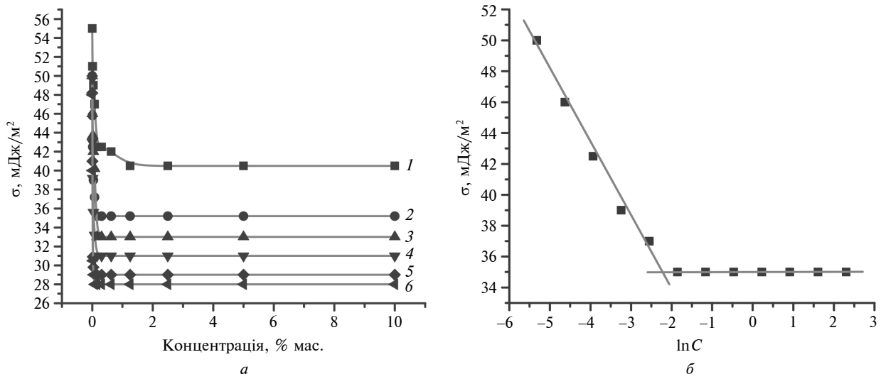
Рис. 1. Залежність поверхневого натягу водних розчинів Tween-80 (1), РБК (6) та їх сумішей від їх загальної концентрації (масовий вміст РБК у суміші, %: 2 – 11,1; 3 – 25,0; 4 – 42,9; 5 – 66,7 (а) та визначення ККМ суміші з 88,9 % Tween-80 і 11,1 % РБК (б)
