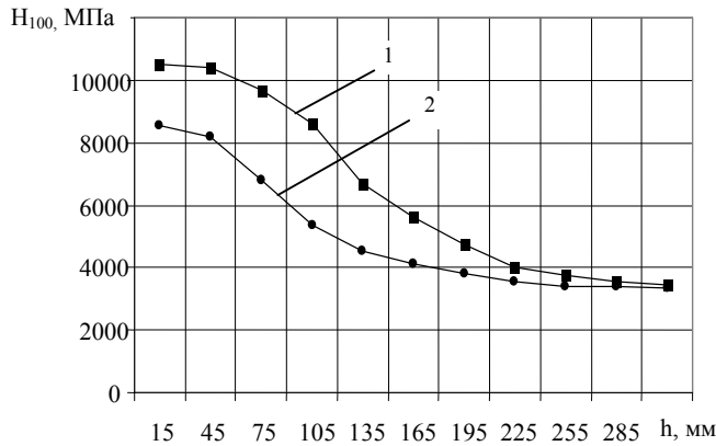
Рис. 2. Зміна мікротвердості по товщині азотованого шару: 1 – ТО + ГТЦ ІА (80%N 2 +5%С 3 Н 8 + 5%Ar; T=600°C; P=175 Па; t=2,5 год); 2 – ГТЦ ІА (80%N 2 +5%С 3 Н 8 +5%Ar; T=600°C; P=175 Па; t=2,5 год)
