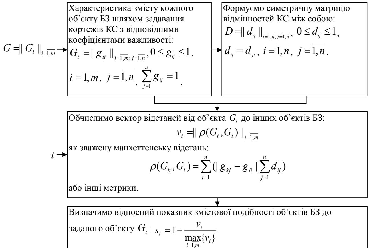
Рис. 2. Метод визначення змістової подібності об'єктів БЗ експертних СППР.
