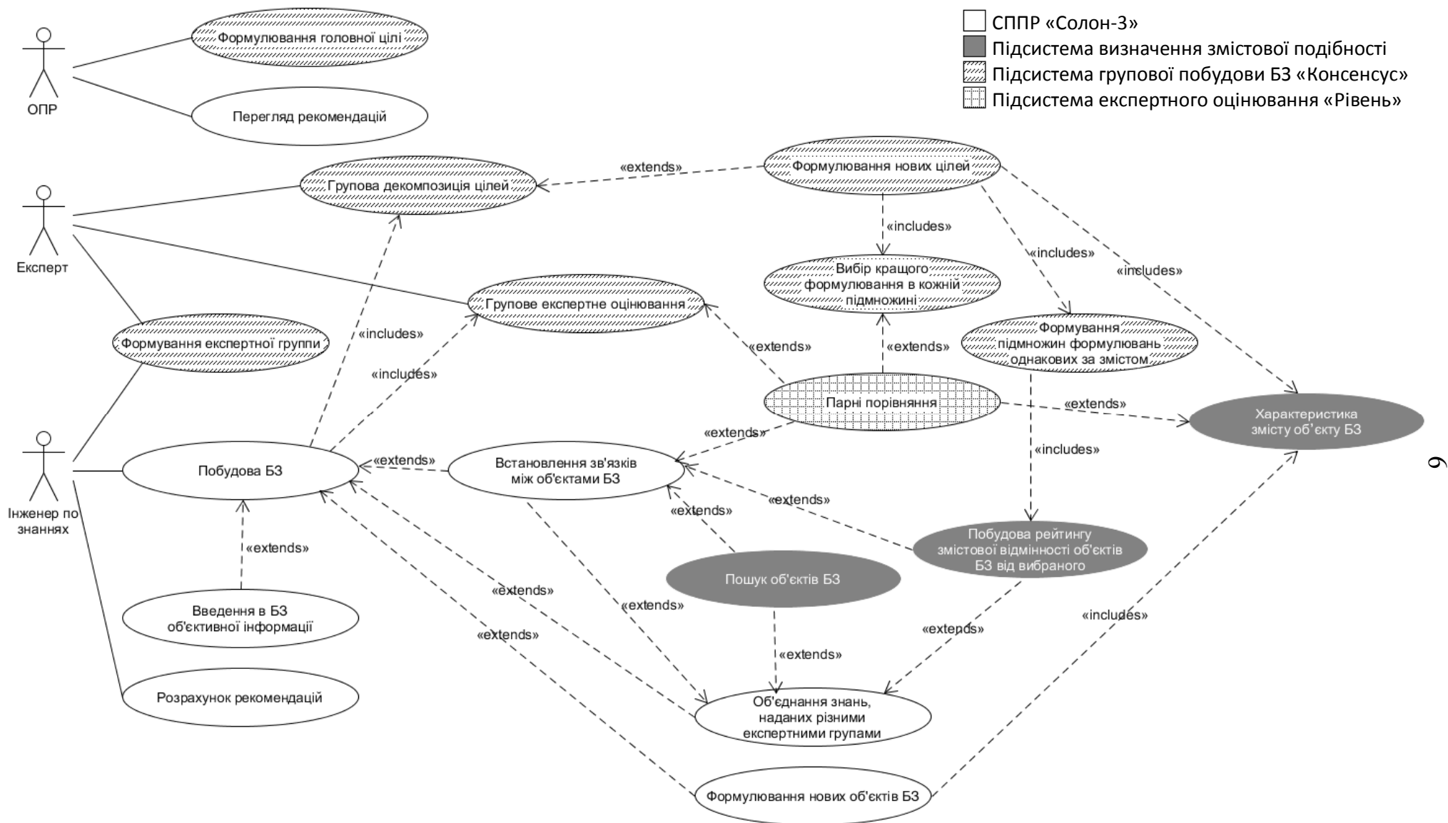
Рис. 1. Use Case діаграма експертної СППР.
