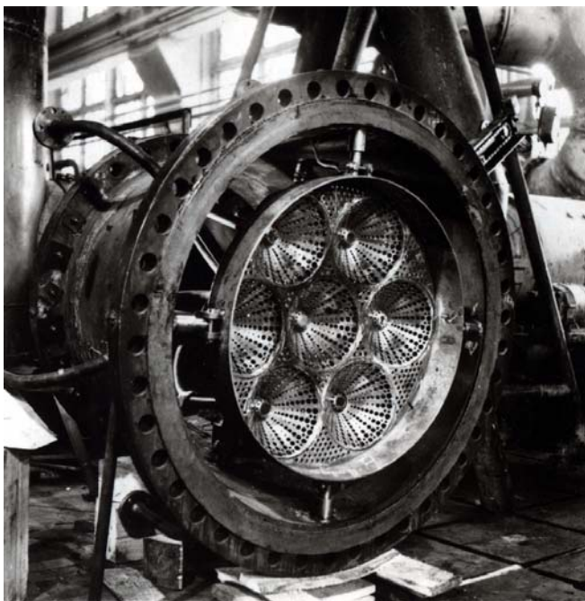
7-модульное фронтное устройство камеры сгорания энергетической ГТУ с струйными горелочными устройствами разработки КПИ
