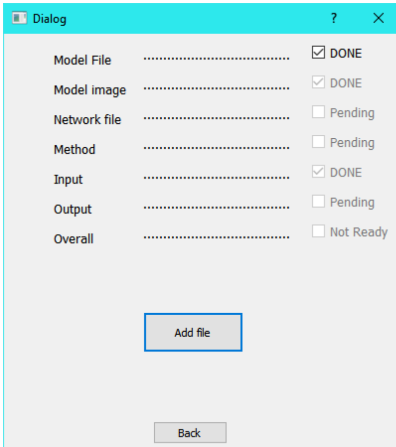
Рисунок 5.3 – Додання файлу
