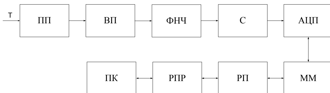
Рис. 1. Структурна схема інформаційно-вимірювальної системи на базі мікроконтролерного модуля:
