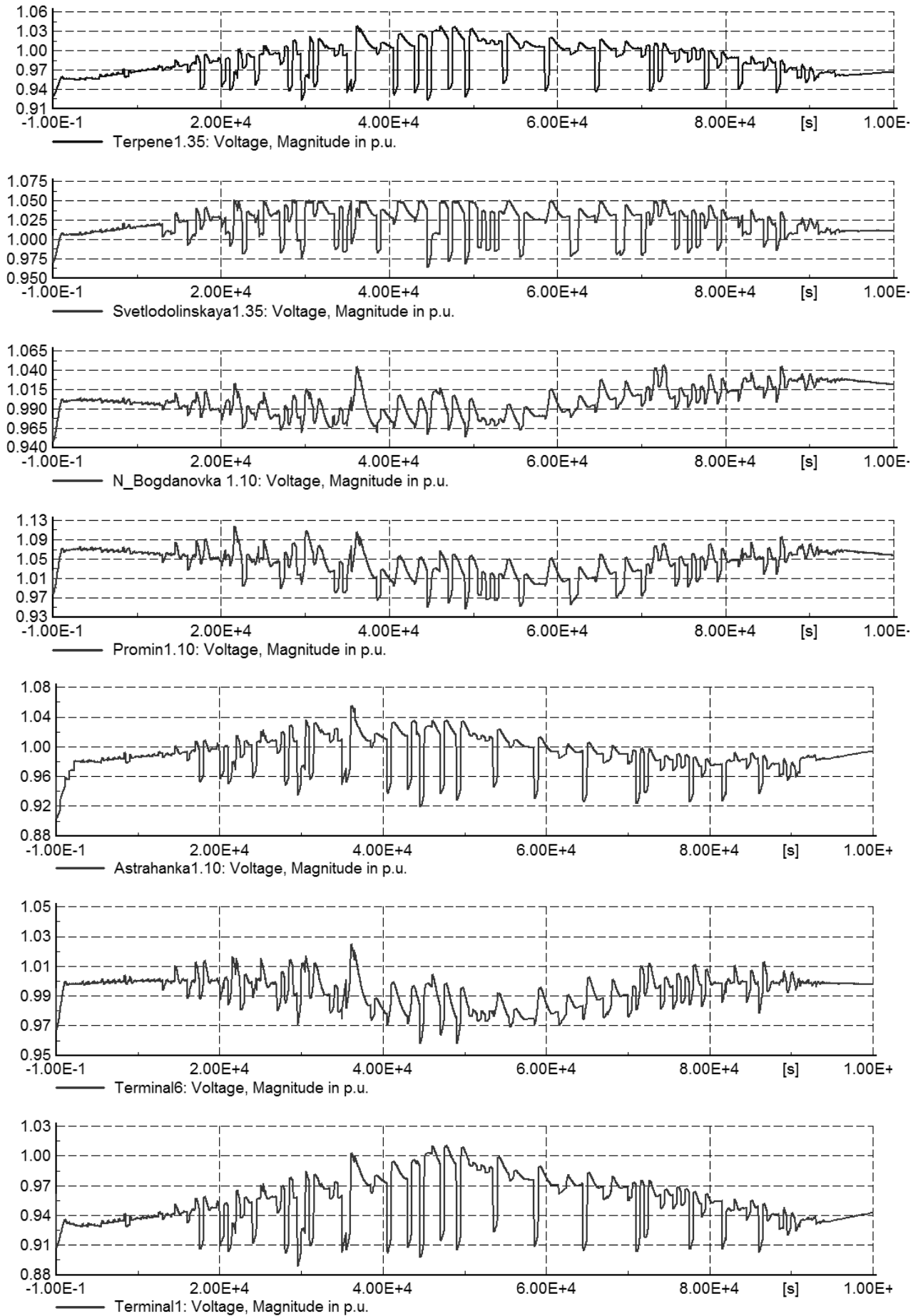
Рисунок Е.9, аркуш 2
