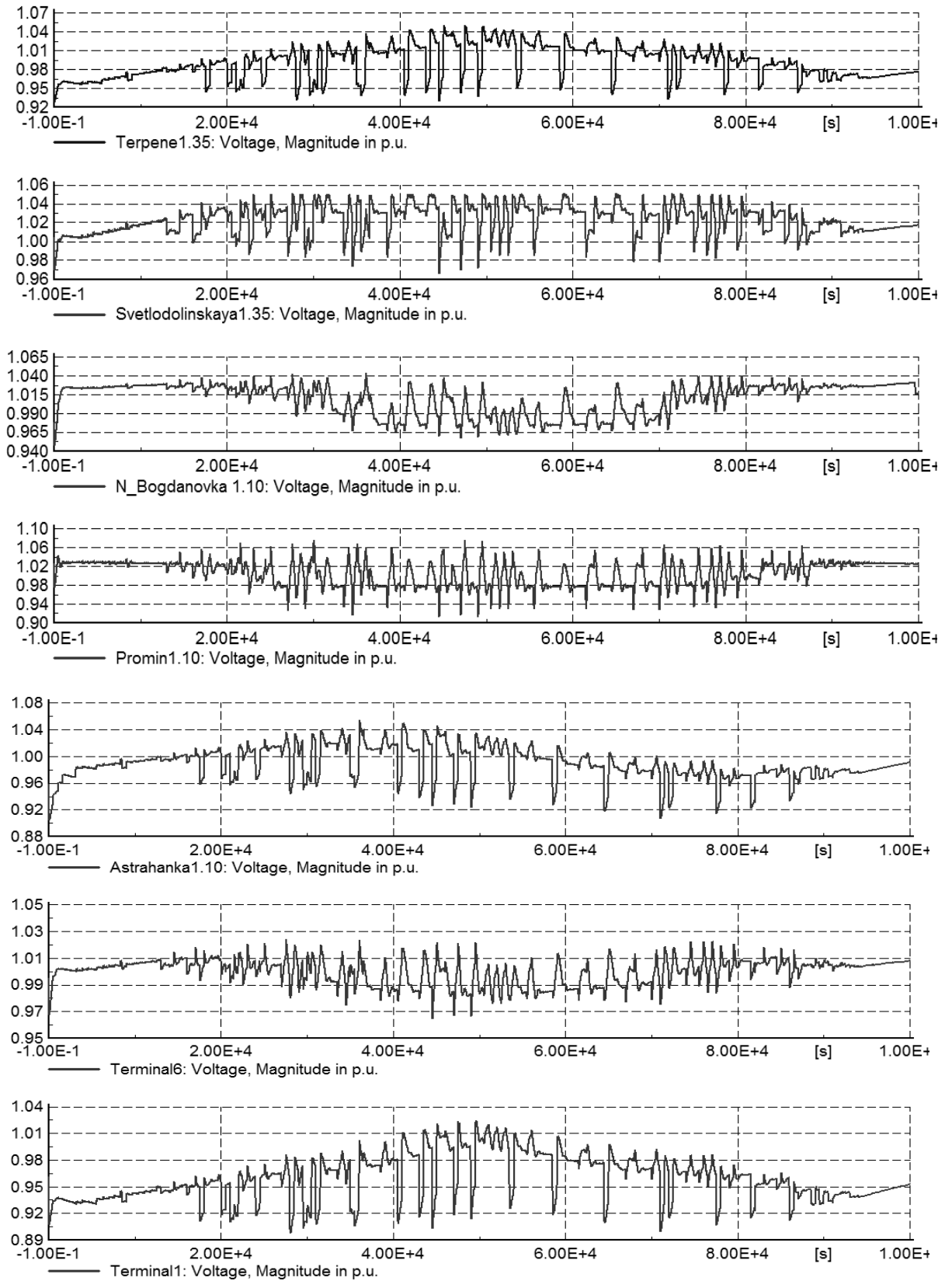
Рисунок Е.9, аркуш 3
