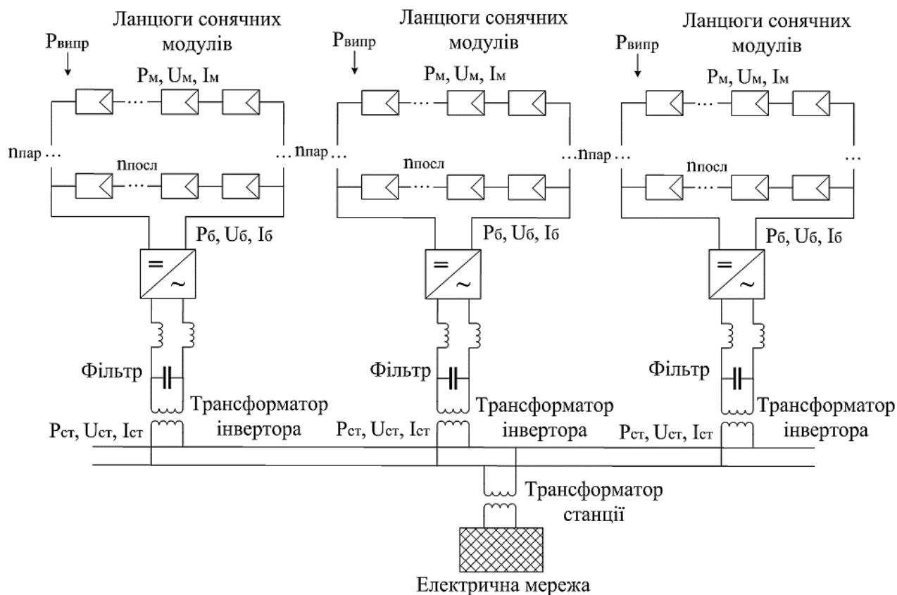
Рисунок 2.9 – Модель фотоелектричної СЕС
