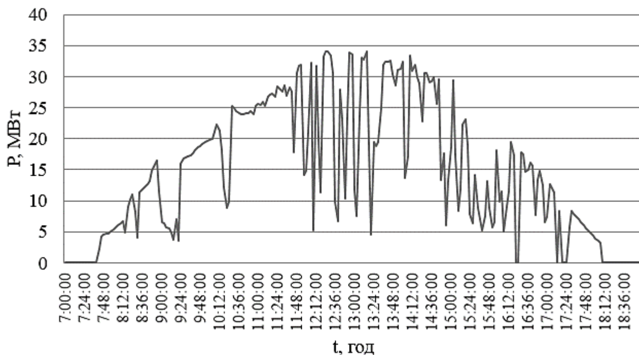
Рисунок 1.5 – Зміна генерації активної потужності СЕС «Дунайська» Одеської енергосистеми за 20.09.2016р.
