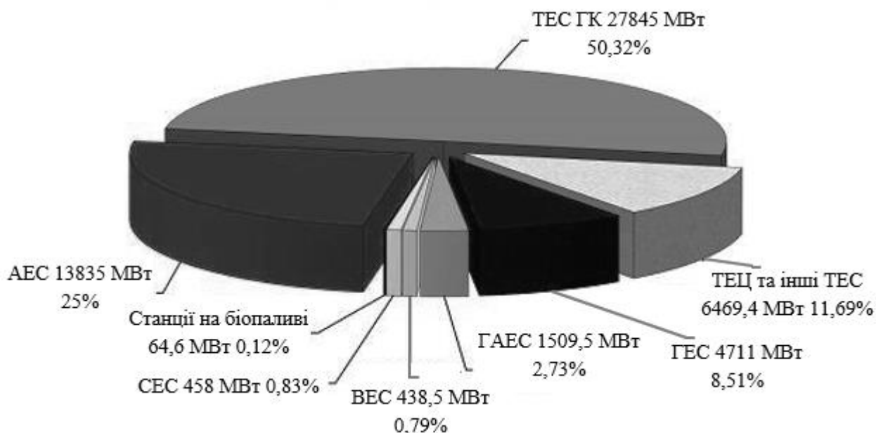
Рисунок 1.4 – Частка генерування ВЕС та СЕС від встановленої потужності ОЕС України станом на 31 грудня 2017 року
