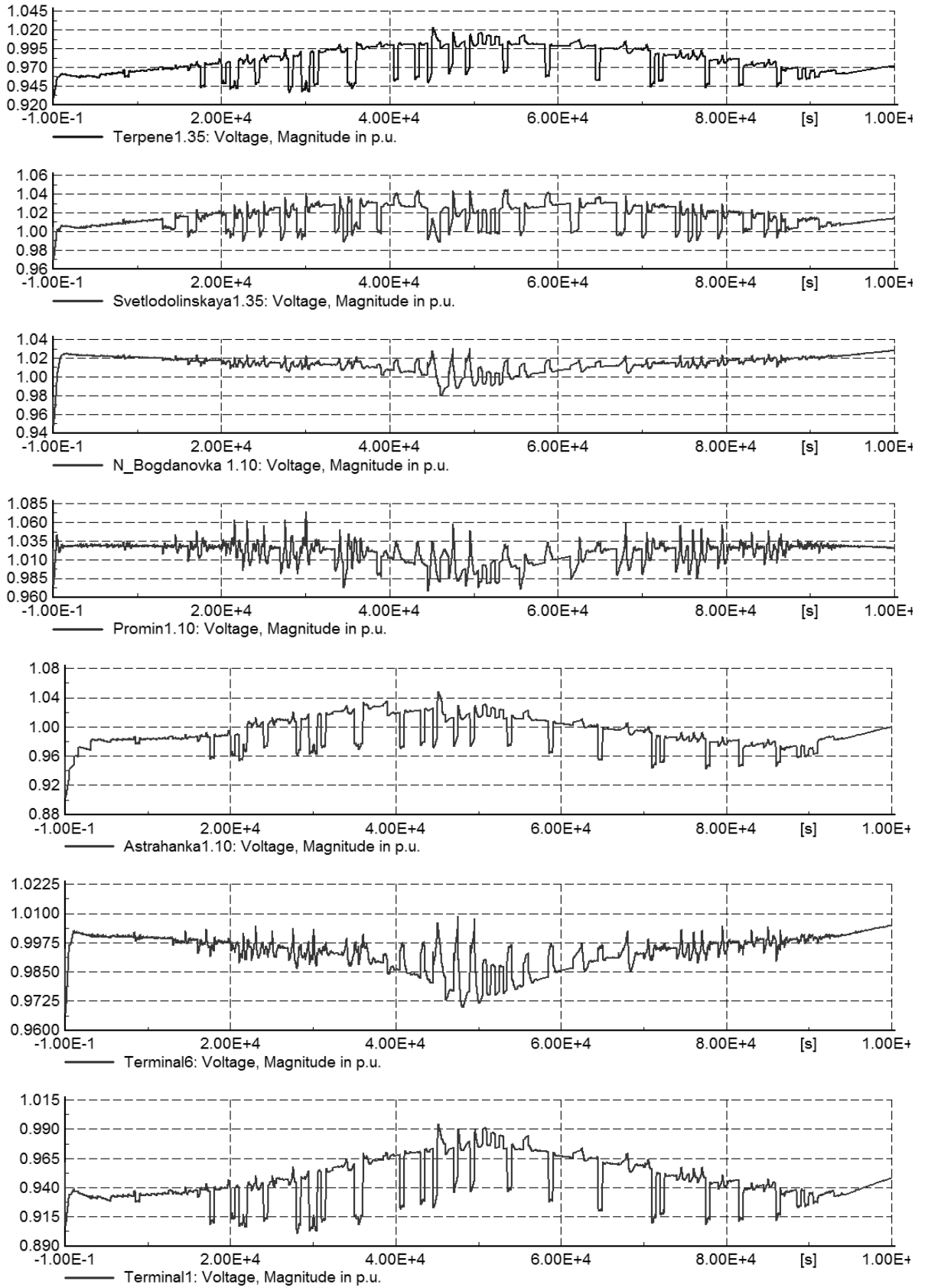
Рисунок Е.10, аркуш 3
