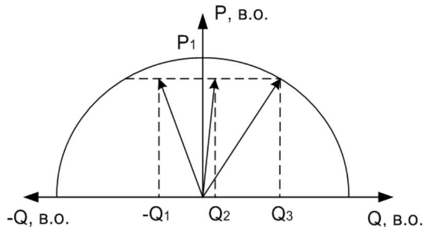
Рисунок 1.10 – Характеристика потужності ДРГ в режимі регулювання реактивної потужності
