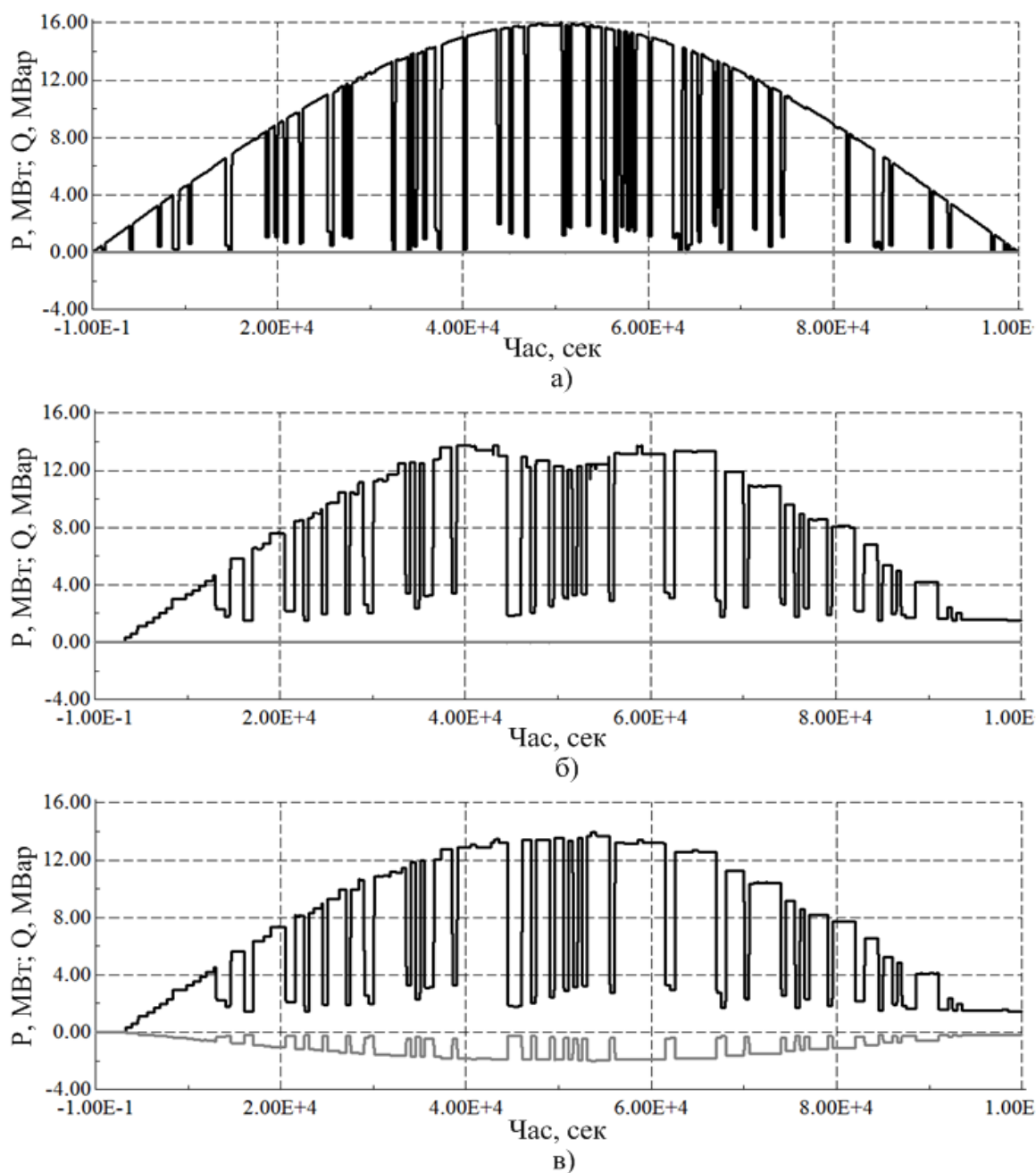
а) без регулювання ДРГ; б) ДРГ працює в режимі регулювання напруги; в) ДРГ працює в режимі регулювання коефіцієнта потужності
