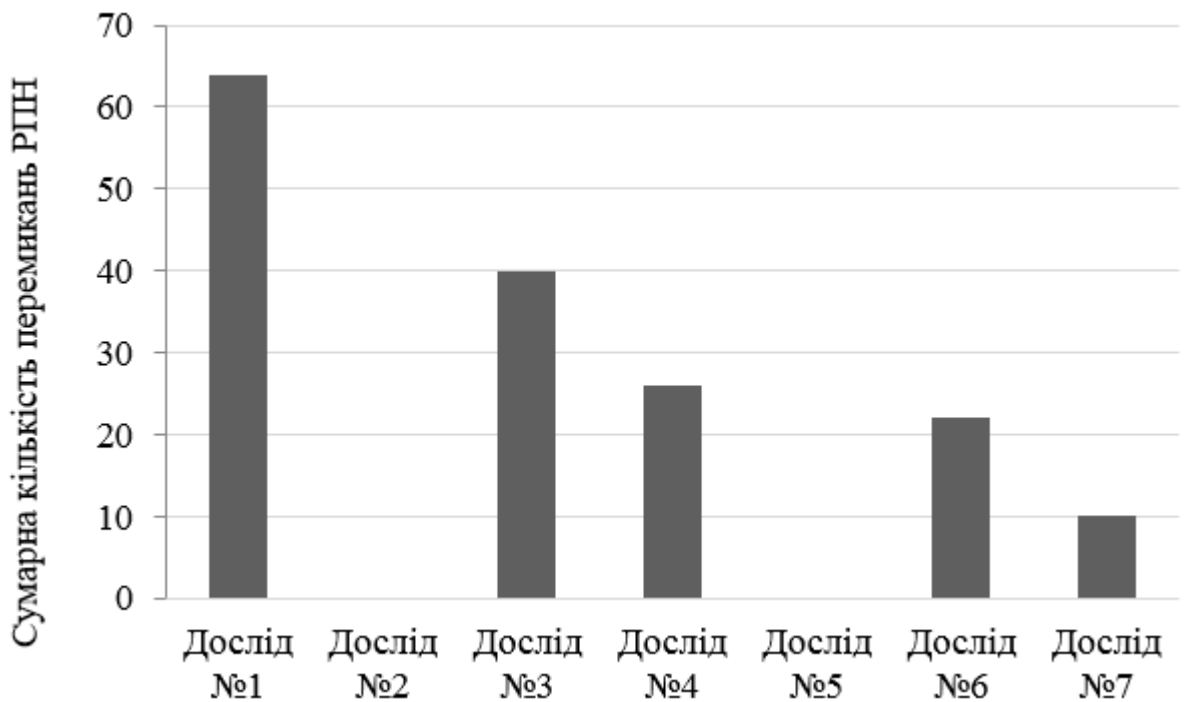
Рисунок 3.8 – Сумарна кількість перемикань положення РПН трансформаторів
