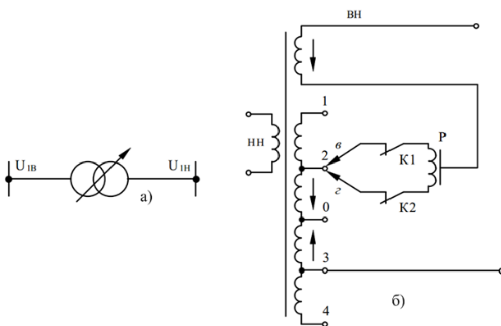
Рисунок 2.3 – Трансформатор з РПН
