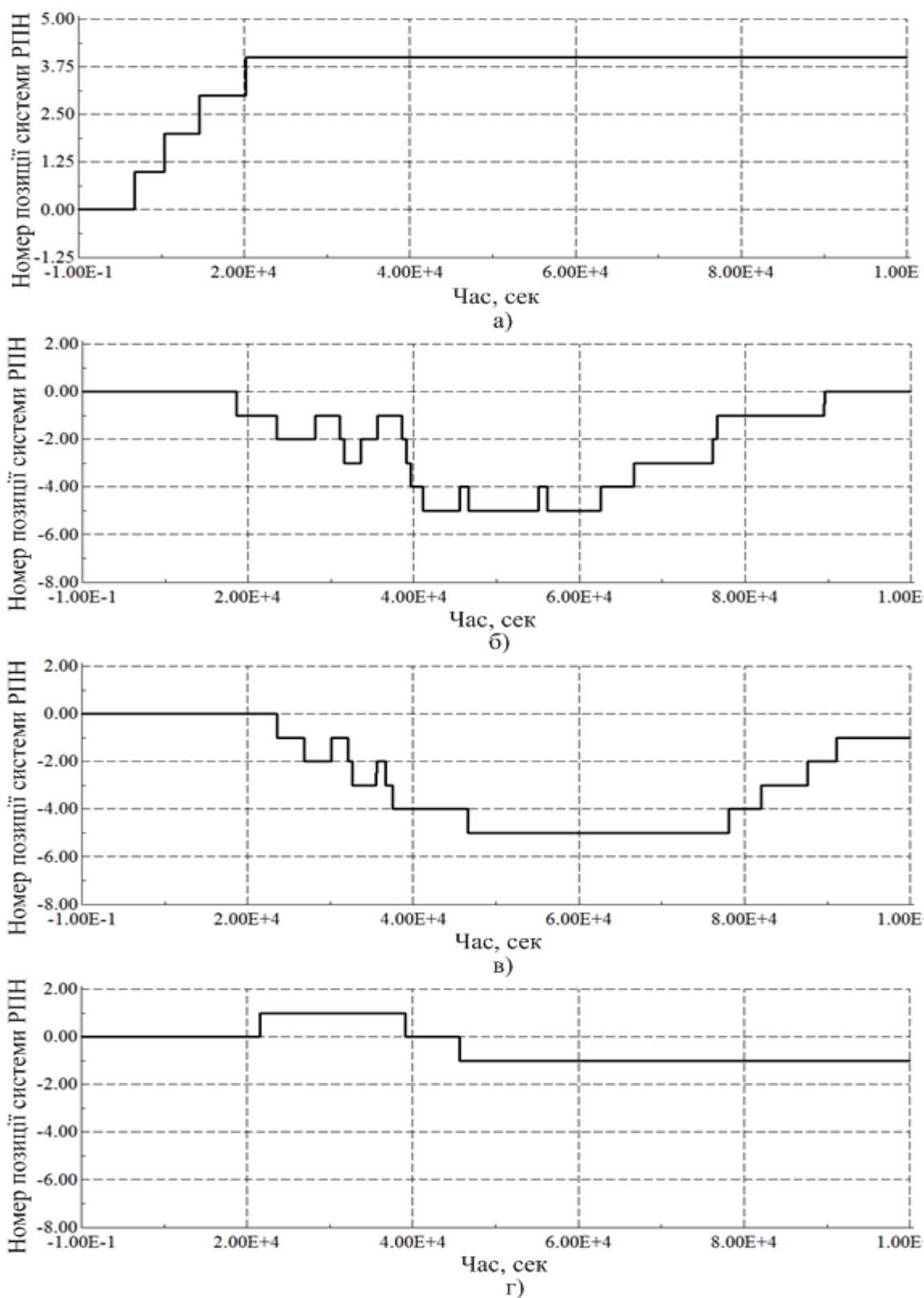
Рисунок 2.21 – Перемикання положення РПН трансформатора при зміні генерування ДРГ протягом доби
