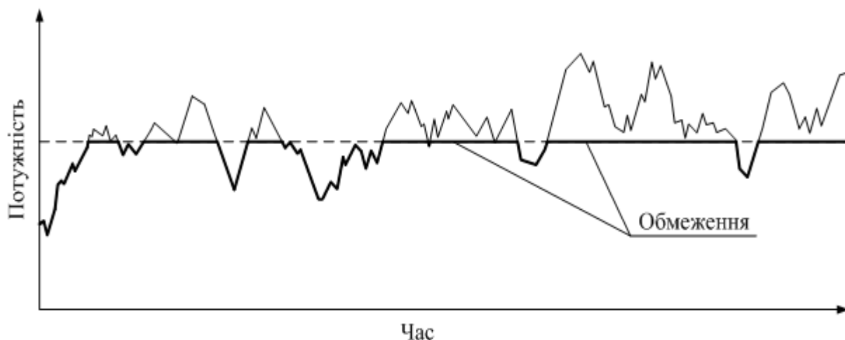
Рисунок 1.13 – Обмеження вихідної активної потужності ДРГ
