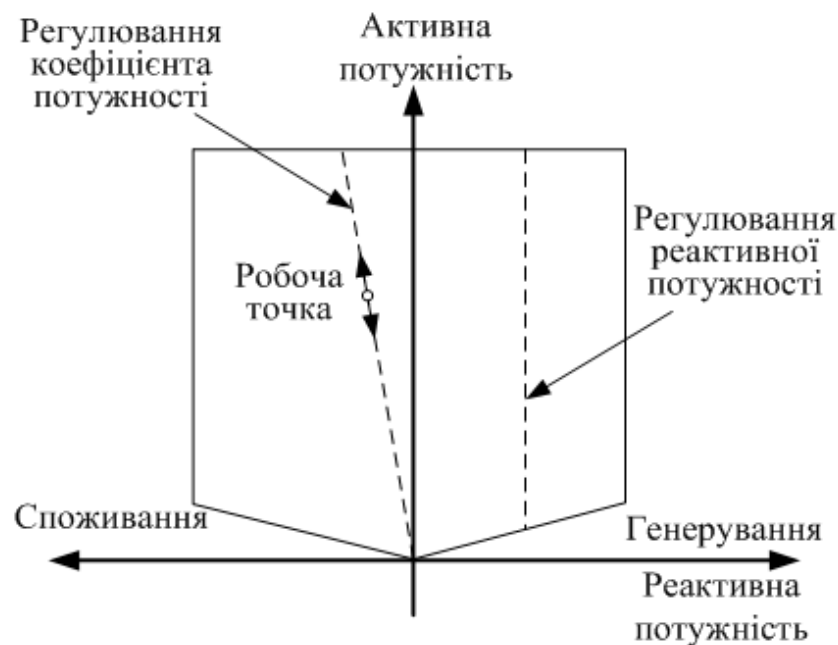
Рисунок 1.8 – Функції регулювання реактивної потужності та коефіцієнта потужності
