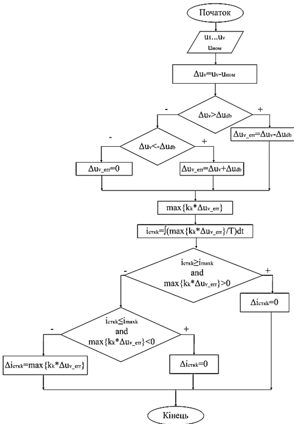
Рисунок 2.15 – Алгоритм роботи підсистеми регулювання реактивної потужності СТК
