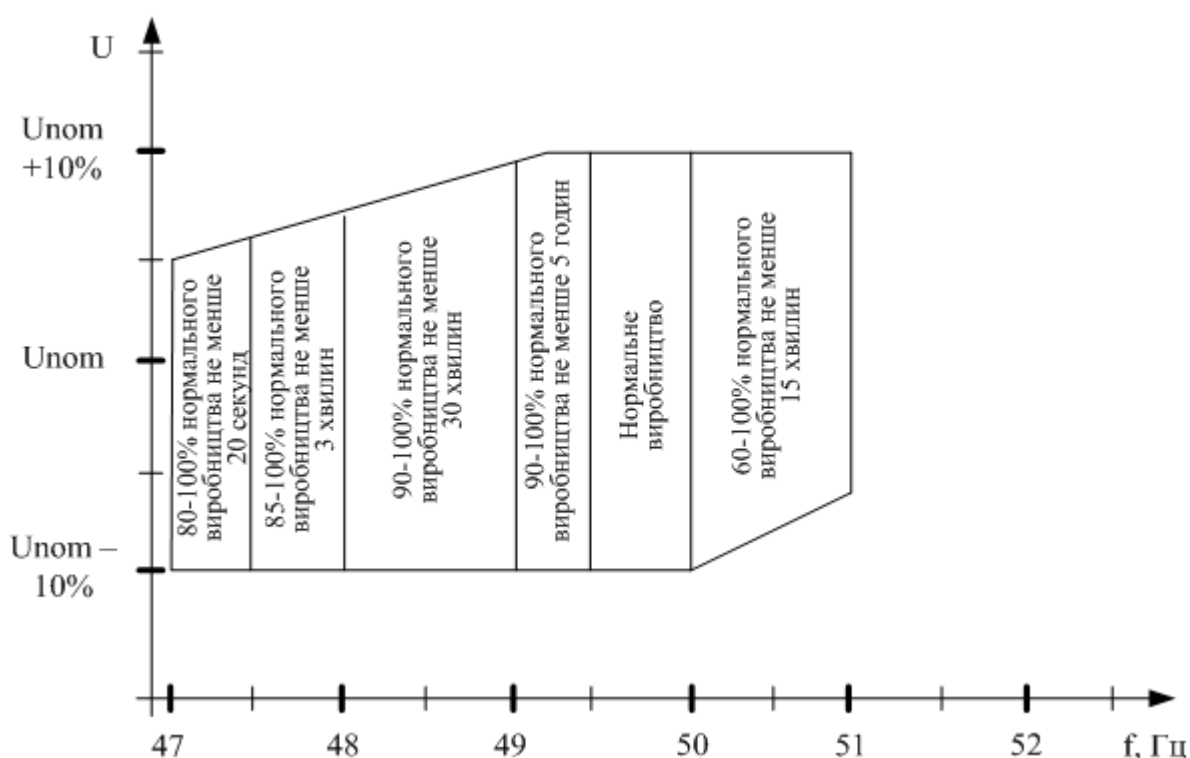
Рисунок 1.7 – Вимоги до генерації активної потужності ДРГ при змінах частоти/напруги
