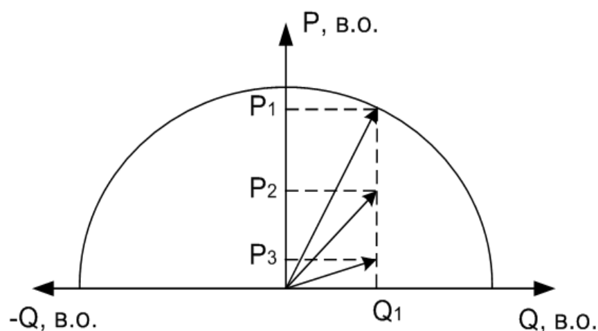
Рисунок 1.11 – Характеристика потужності ДРГ з фіксованим значенням реактивної потужності
