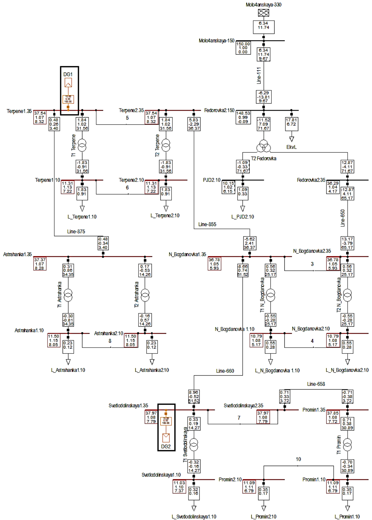
Рисунок 2.17 – Фрагмент РЕМ 110/35/10 кВ Молочанського району Запорізької області
