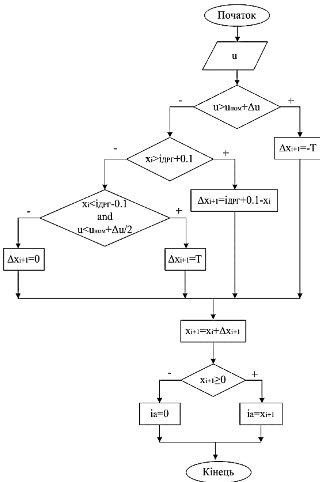
Рисунок 2.13 – Алгоритм роботи підсистеми керування потужністю ДРТ в режимі регулювання напруги
