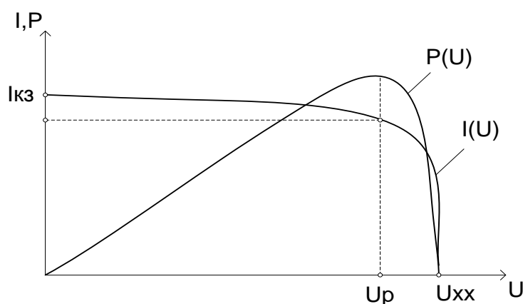
Рисунок 2.10 – Вольт-амперна характеристика фотоелектричного модуля
