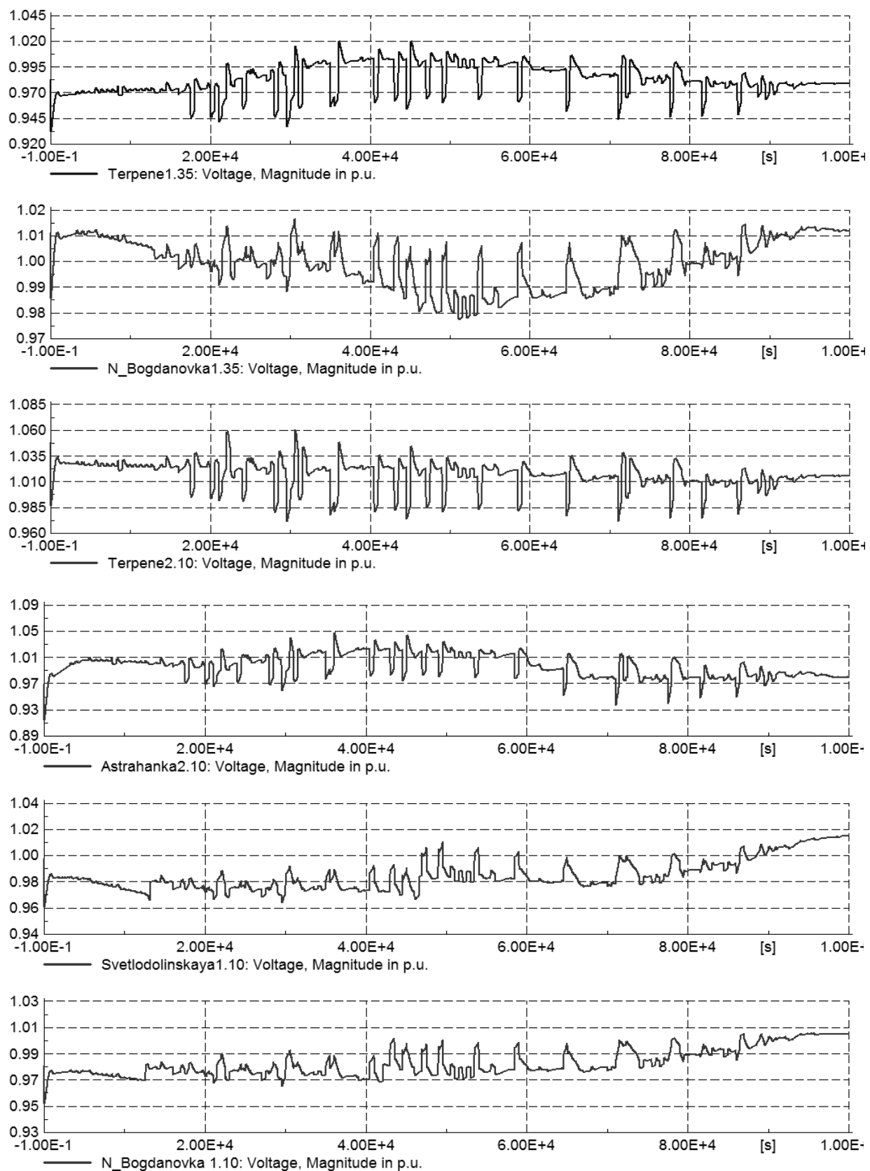
Рисунок Е.6, аркуш 3
