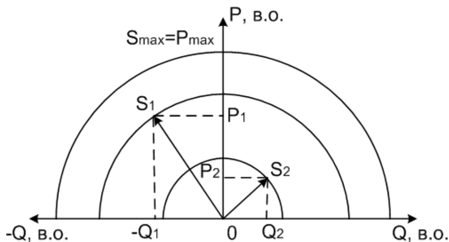
Рисунок 1.12 – Характеристика потужності ДРГ в режимі регулювання напруги
