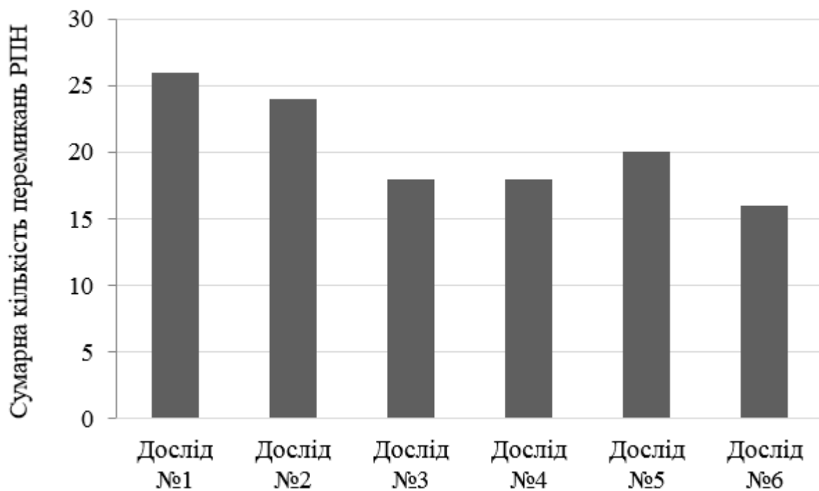
Рисунок 4.13 – Сумарна кількість перемикачів положення РПН трансформаторів
