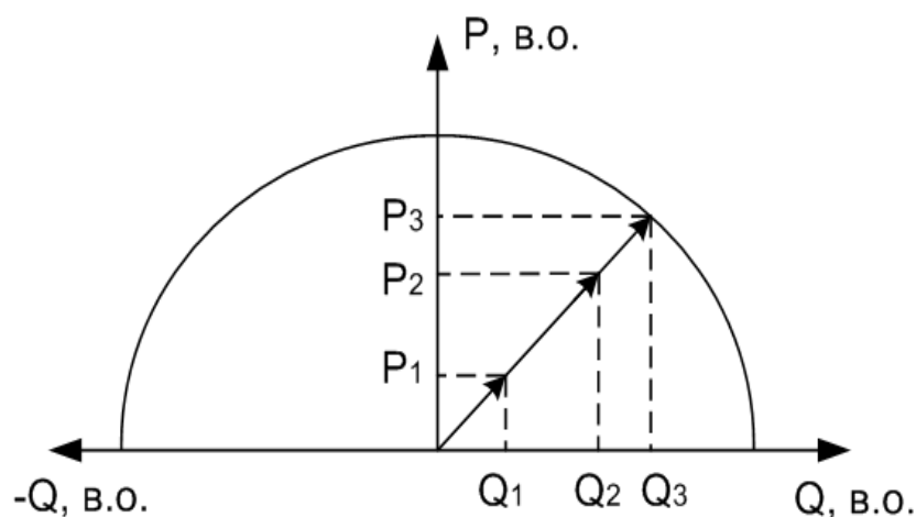
Рисунок 1.9 – Характеристика потужності ДРГ в режимі регулювання \cos\varphi
