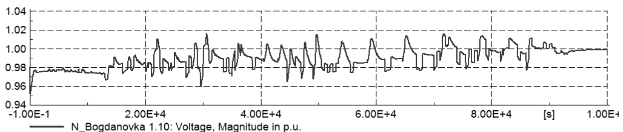
Рисунок Е.5, аркуш 3
