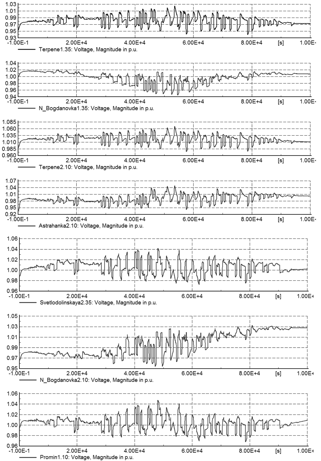
Рисунок Е.8, аркуш 2
