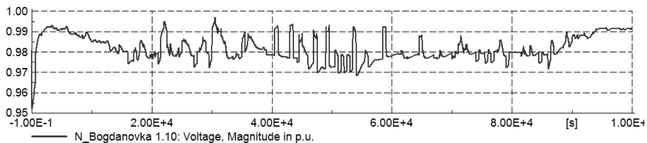
Рисунок Е.6, аркуш 2
