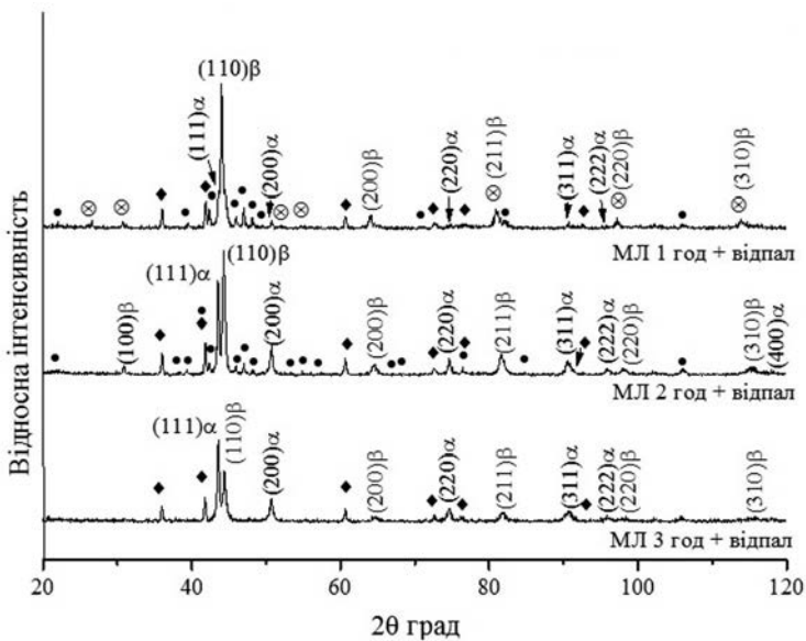
Рис. 3. Спектри рентгенівської дифракції порошкового AlNiCoFeCrTi сплаву після механічного легування (1, 2 та 3 год) та гомогенізуючого відпалу, 1200 °С, 1 год.
