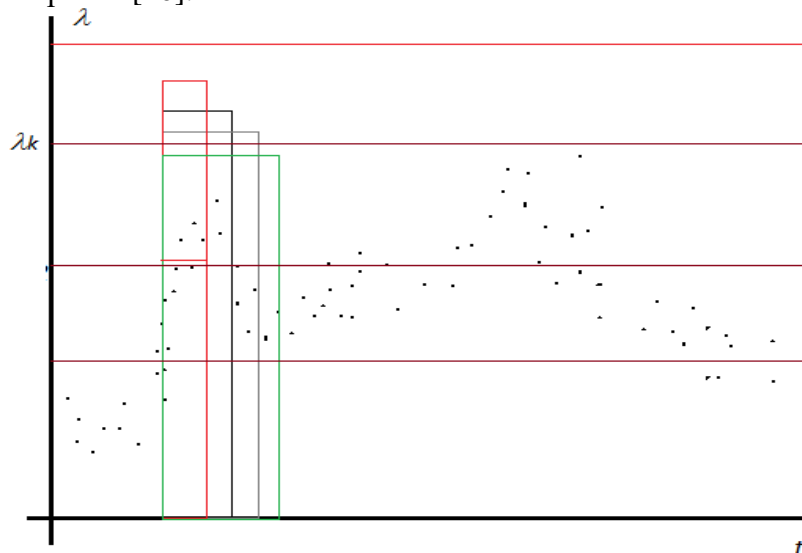
Рис. 2. Метод побудови розкладу вибору конфігурацій на основі довгострокової статистики
