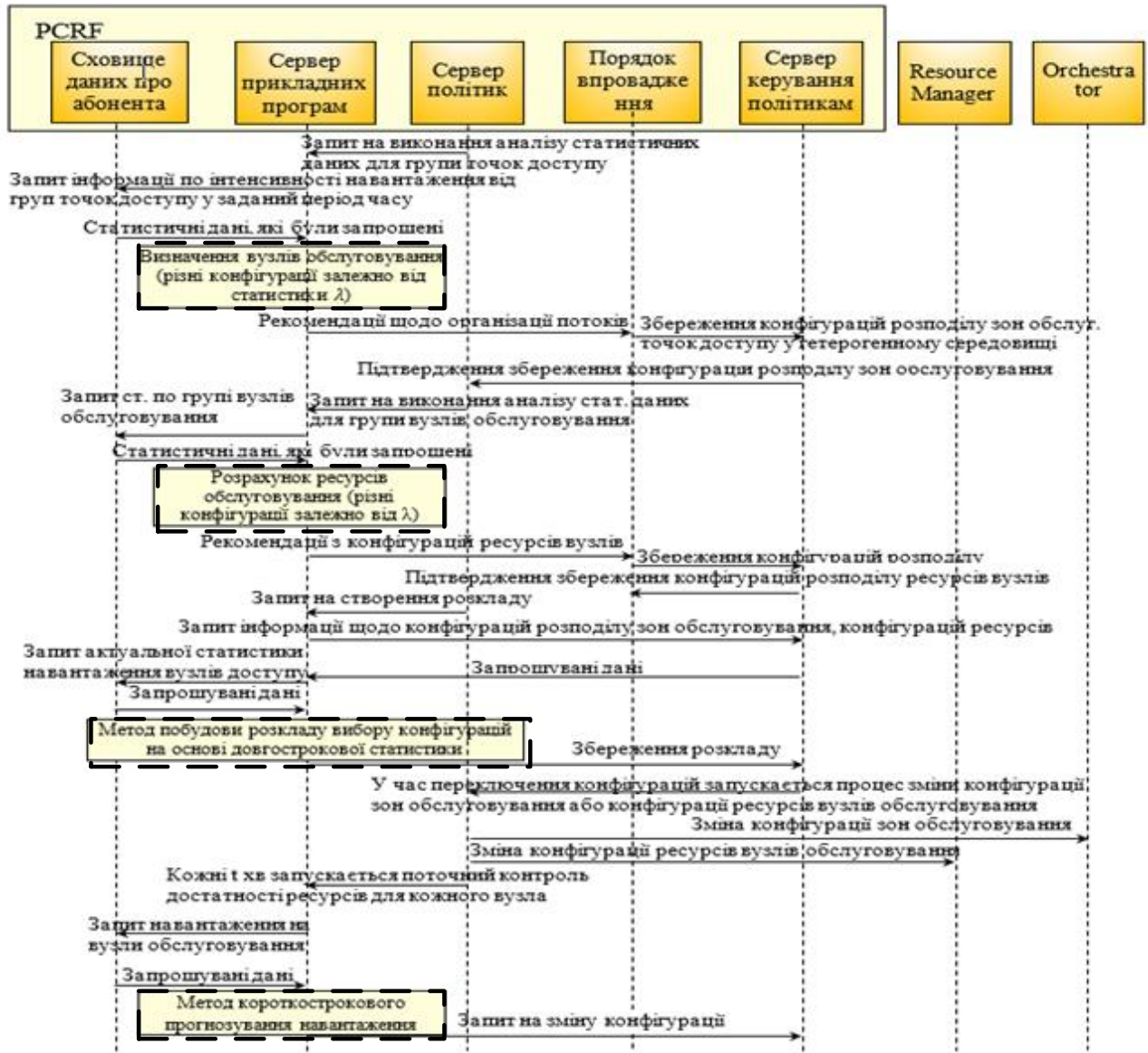
Рис.4. Процедура планування обсягу ресурсів гетерогенного телекомунікаційного середовища
