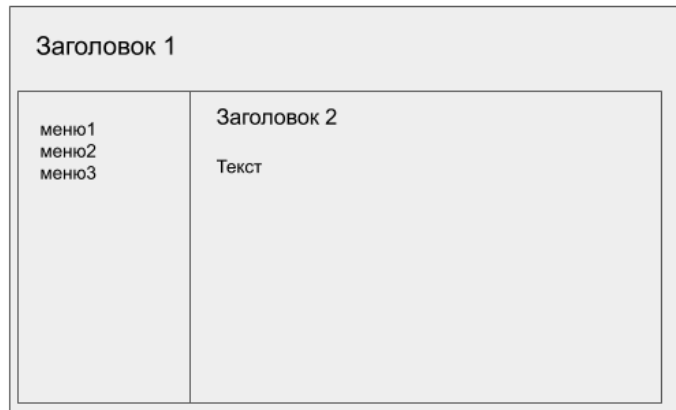
Рис. 2.1. Шаблон HTML-документу
