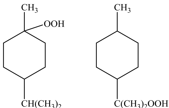
Гідроперокси ментану (4-ізопропіл-1-метилциклогексану)
