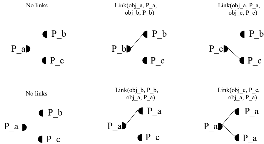
Рисунок 4.1 – Встановлення зв'язків між позиціями Петрі-об'єктів:
