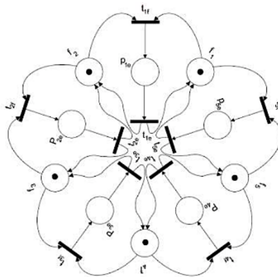
Рисунок 5.11 – Модель «філософів», представлена стохастичною мережею Петрі [54].
