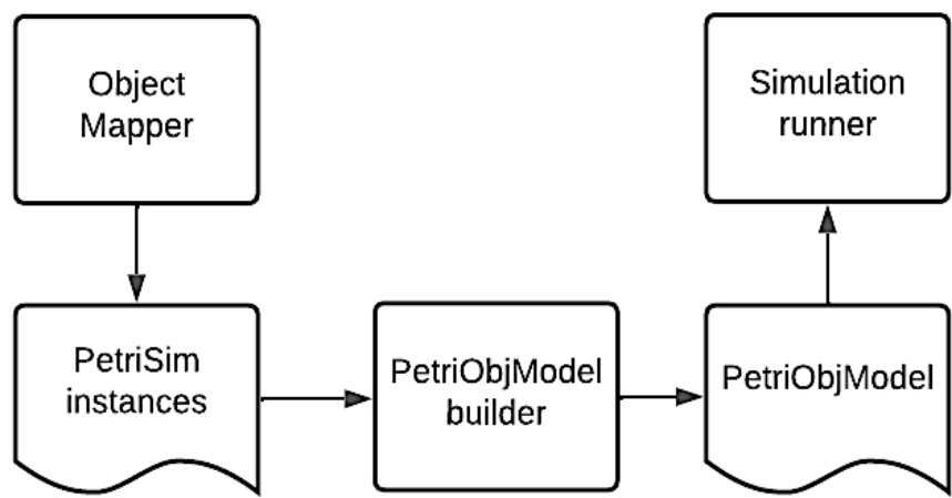
Рисунок 4.3 – Серверна частина транслятора
