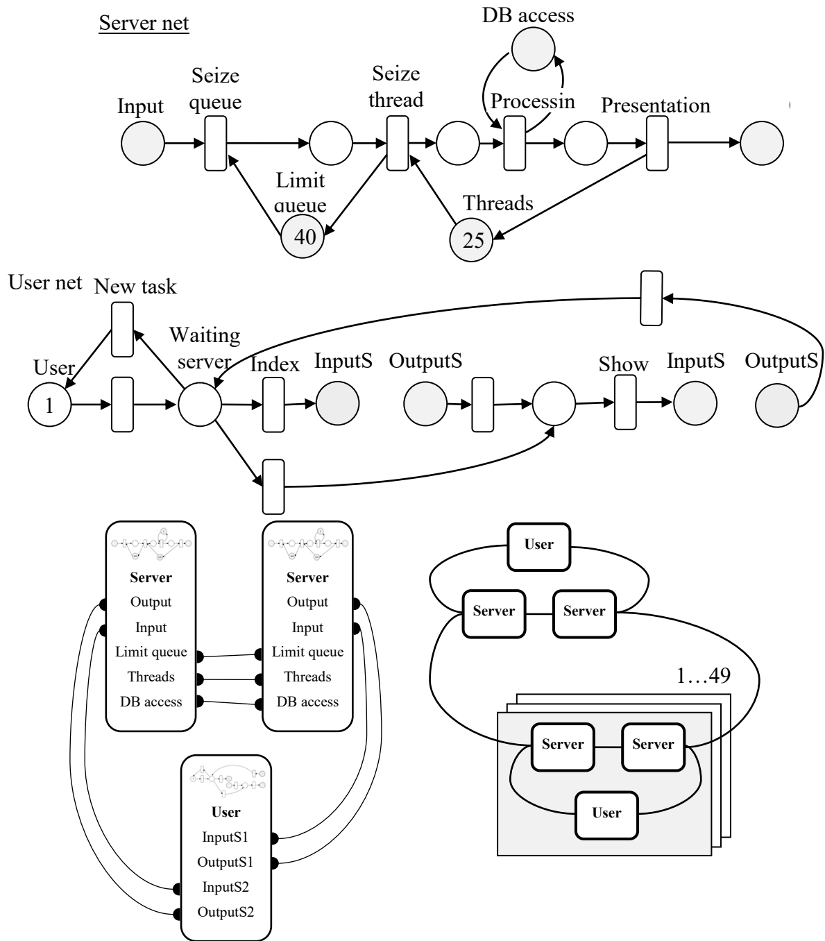
Рисунок 3.2 - Фрагмент Петрі-об'єктної моделі інформаційної системи, розроблений мовою візуального програмування
