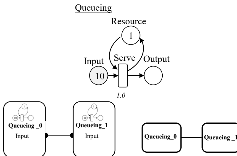
Рисунок 5.3 – Модель, що складається з одного триплета Петрі-об'єкт – конектор – Петрі-об'єкт.
