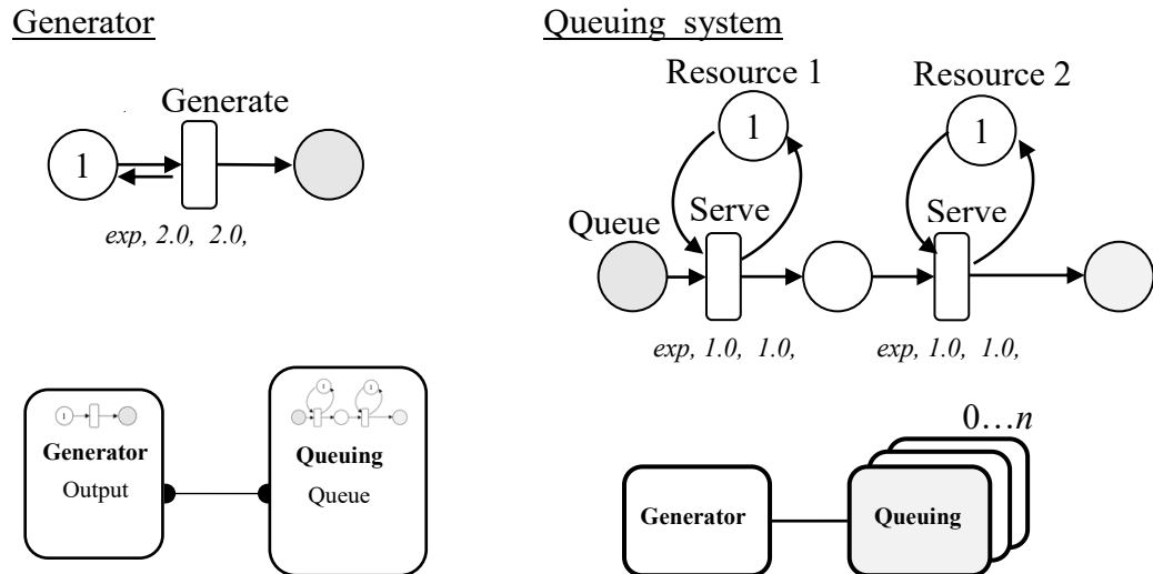
Рисунок 4.4 – Візуальне представлення Петрі-об'єктної моделі масового обслуговування: мережі Петрі-об'єктів, ототожнення позицій Петрі-об'єктів, триплет об'єкт-конектор-група.
