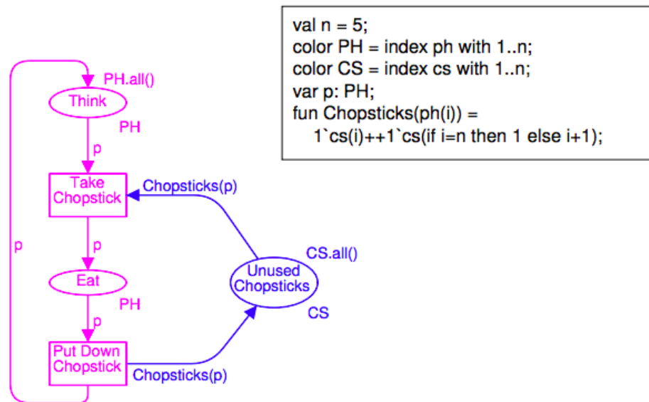
Рисунок 5.12 – Модель «філософів», представлена розфарбованою мережею Петрі [55].
