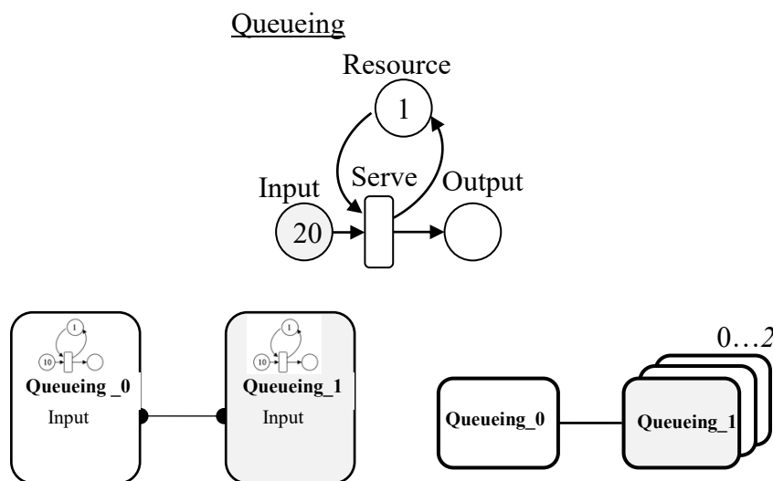
Рисунок 5.5 – Модель, що складається з одного триплета Петрі-об’єкт – конектор – група Петрі-об’єктів.
