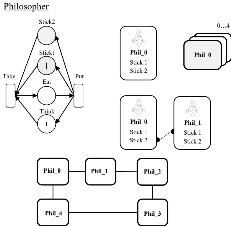
Рисунок 5.13 – Петрі-об’єктна модель «філософів», розроблена мовою візуального програмування
