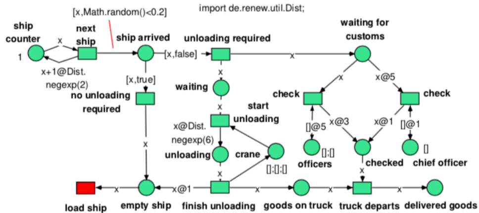
Рисунок 1.3 – Візуальне представлення мережі Петрі в редакторі Renew 4.0 [16]
