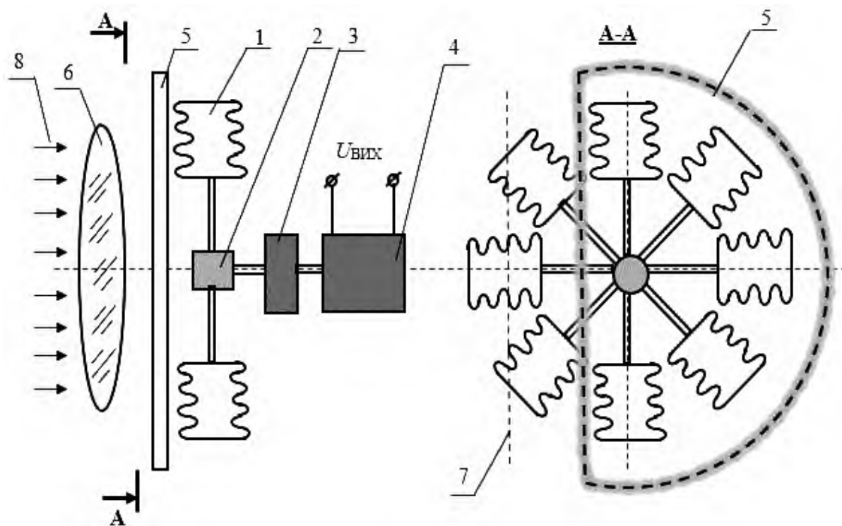
Схема установки пневмо-оптичного генератора електричної енергії:
