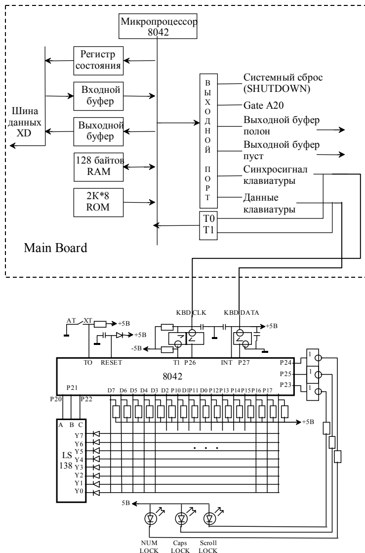
Рисунок 1 – Блок-схема контроллера клавиатуры
