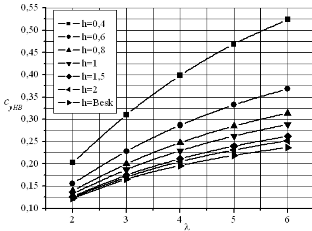
Рис. 10. Залежності c_{yHB} = f(\lambda) трапецевидного крила при різних
