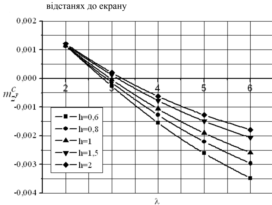
Рис. 9. Залежності m_z^C = f(\lambda) трапецевидного крила при різних відстанях до екрану
