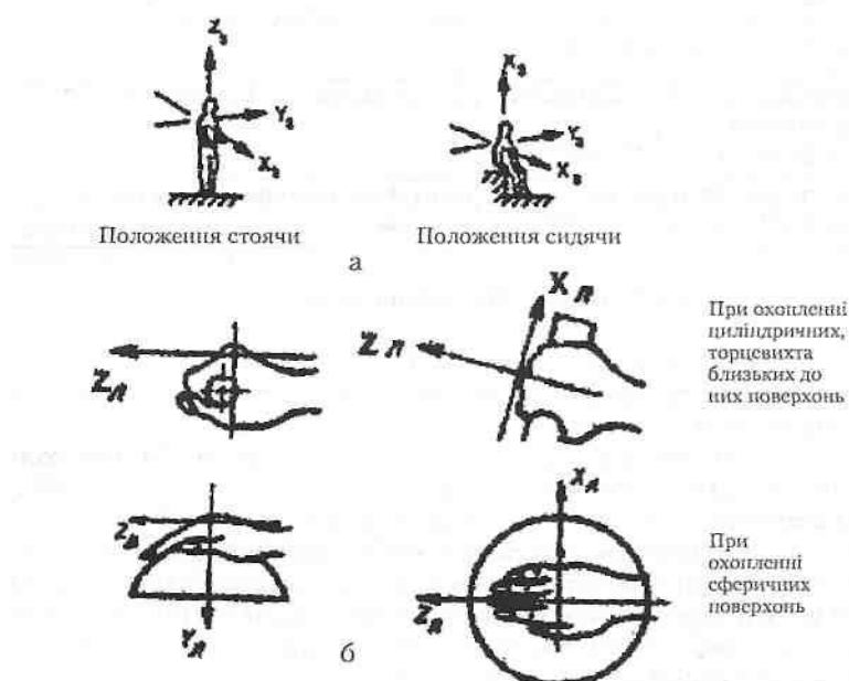
Рис.3.1. Напрями координатних осей: а) дія загальної вібрації; б) дія локальної вібрації
