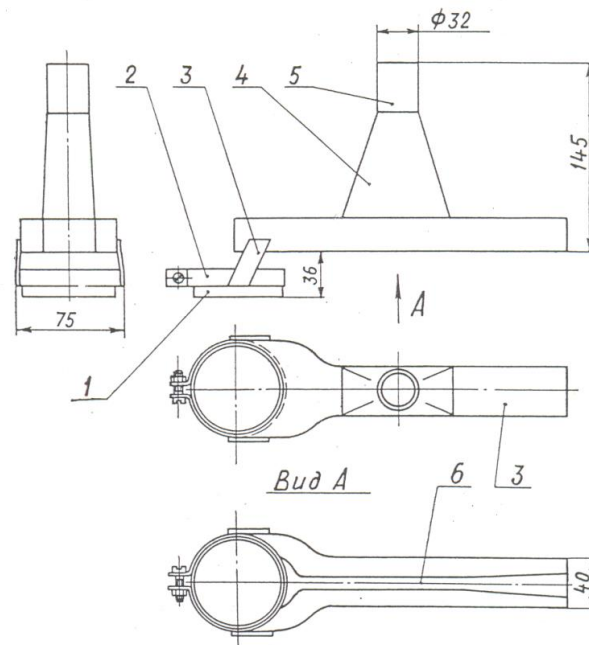
Рис. 3.22. Щілинний відсмоктувач до автомата для зварювання під флюсом (ВЦНДІОП): 1 – кільце; 2 – хомут; 3 – планка; 4 – конфузор; 5 – патрубок; 6 – щілина рівномірного всмоктування
