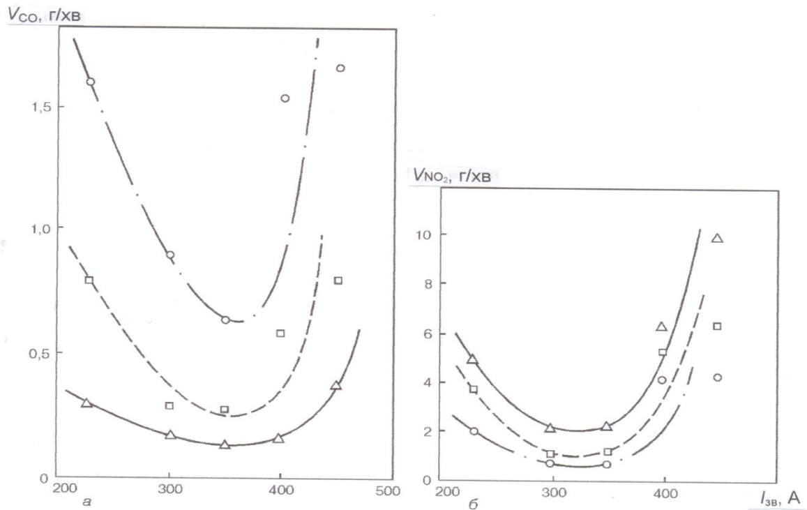
Рис. 3.9. Залежність інтенсивності утворення монооксиду вуглецю V_{CO} (а) і діоксиду азоту V_{NO_2} (б) від сили струму при зварюванні дротом Св-08Г2С діаметром 1,6 мм в захисних газах: \circ – CO_2 ; \square – Ar+CO_2 ; \Delta – Ar+CO_2+O_2
