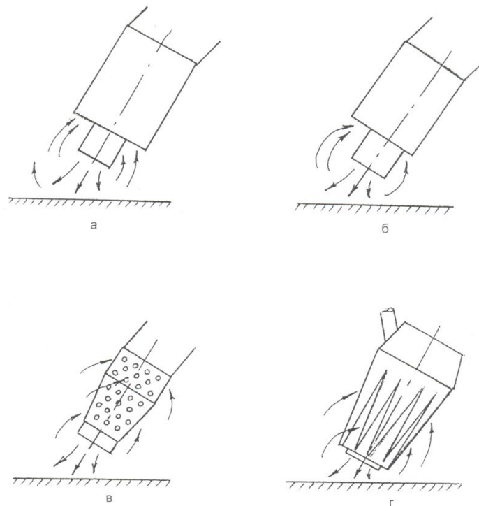
Рис. 3.21. Схеми аспіраційних пристроїв до пальників для напівавтоматичного зварювання в CO_2 : а – циліндричний коаксиальний; б – циліндричний аксиальний; в – конусно-дірчатий коаксиальний; г – конусно-щілинний коаксиальний
