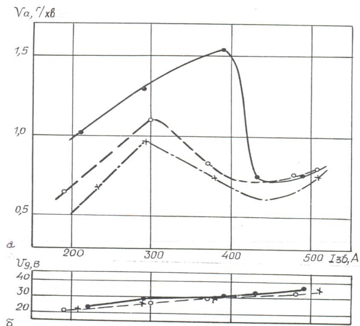
Рис. 3.5. Залежність інтенсивності утворення ЗА V_a від сили зварювального струму (а) і вольт-амперні характеристики дуги (б): ● – зварювання в \text{CO}_2 ; ○ – \text{Ar} + \text{O}_2 + \text{CO}_2 ; x – \text{Ar} + \text{CO}_2 (дріт Св-08Г2С)
