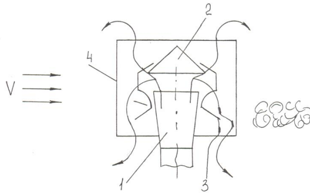
Рис. 3.12. Дефлектор конструкції ЦАГІ: 1 – витяжна труба; 2 – протидощовий ковпак (зонт); 3 – конус, що запобігає зворотній тязі повітря у приміщення; 4 – зовнішня оболонка
