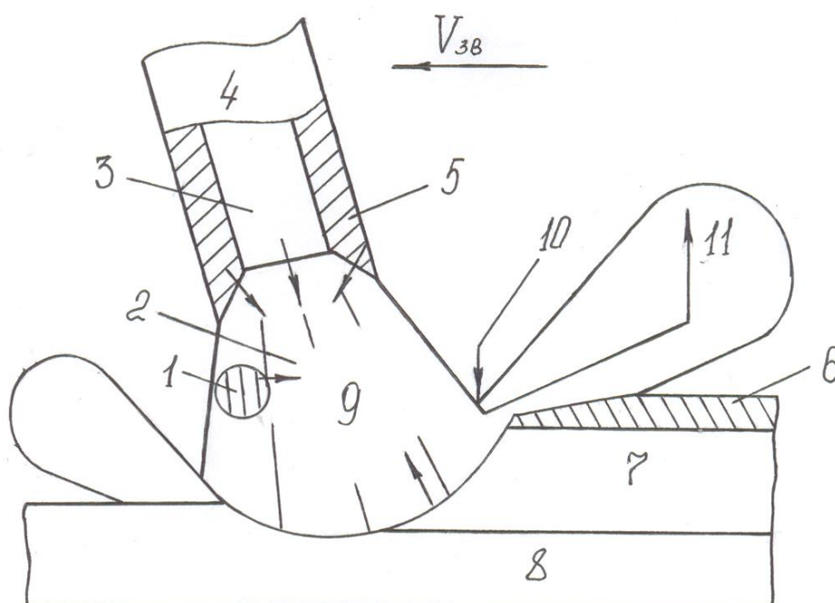
Рис. 3.2. Механізм утворення ЗА при зварюванні покритими електродами: 1 – крапля металу; 2 – дуга; 3 – стрижень електрода; 4 – електрода, що плавиться; 5 – покриття електрода; 6 – шлак; 7 – метал шва; 8 – основний метал; 9 – високотемпературна пара; 10 – границя конденсації; 11 – аерозоль
