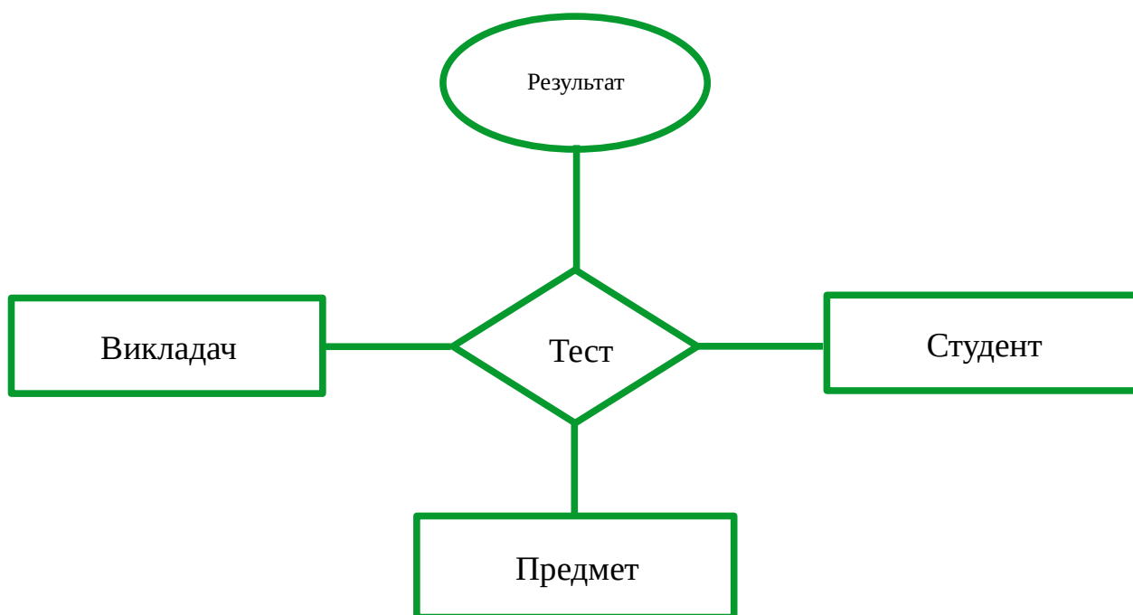
Рис. 2.9.Тернарний зв'язок
