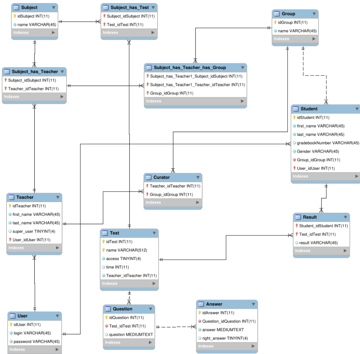
Рис. 3.1. EER діаграма
