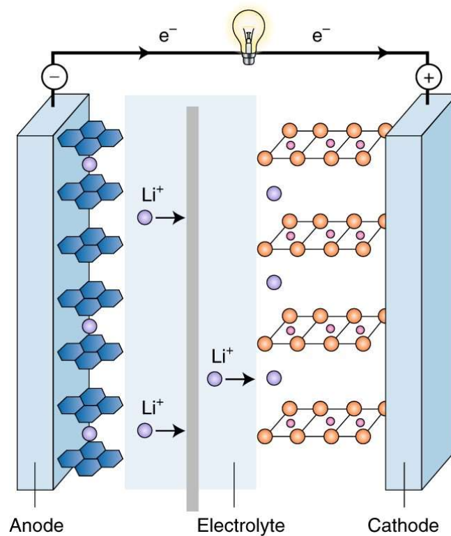
Рис. 5.3. Принцип літій-іонного акумулятора.
