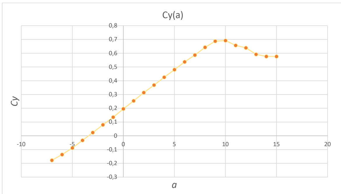
Графік 4.1. Коефіцієнт підйомної сили C_y відносно кута атаки \alpha :
