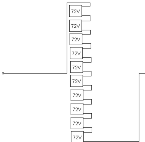
Рис. 7.2. Блок 724V5860W
