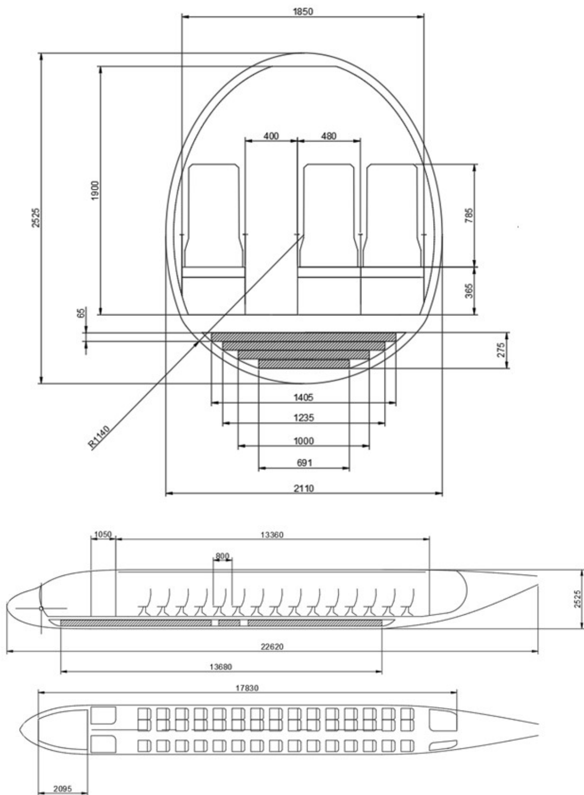
Рис. 3.2. Геометричні параметри фюзеляжу.
