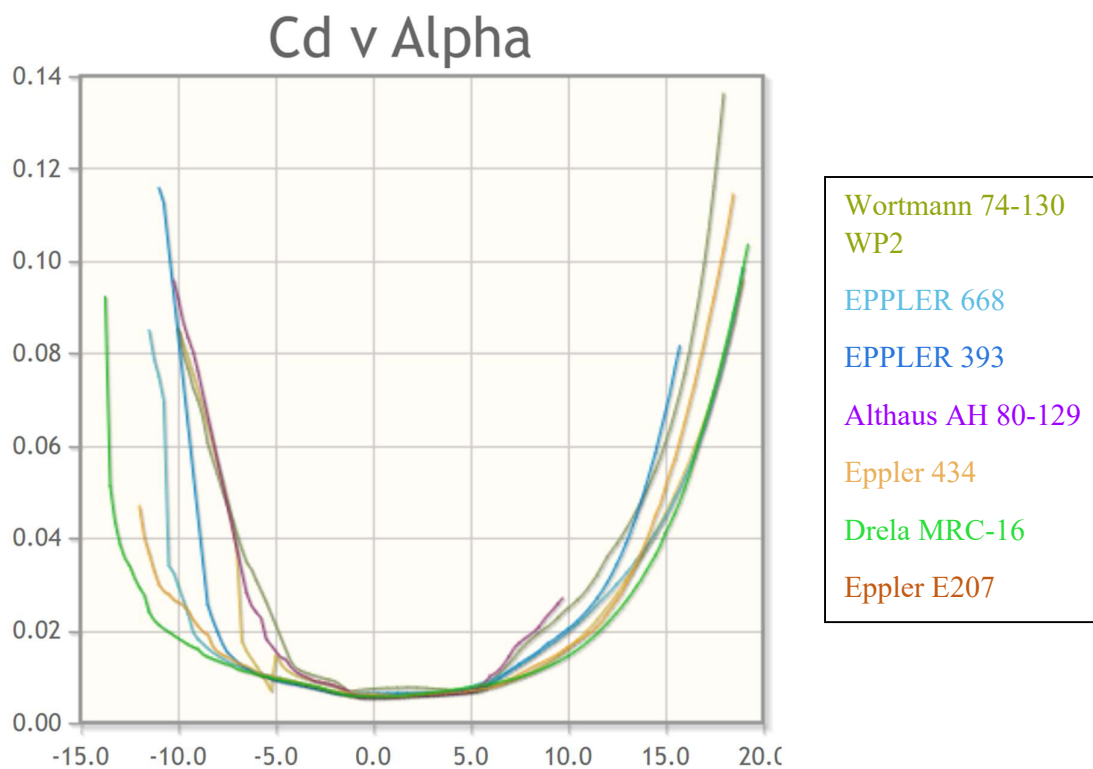
Рис. 3.10. Коефіцієнт лобового опору відносно кута атаки.
