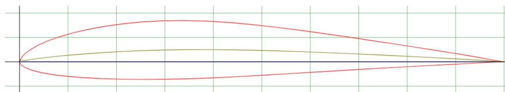
Рис. 3.6. Althaus AH 80-129
