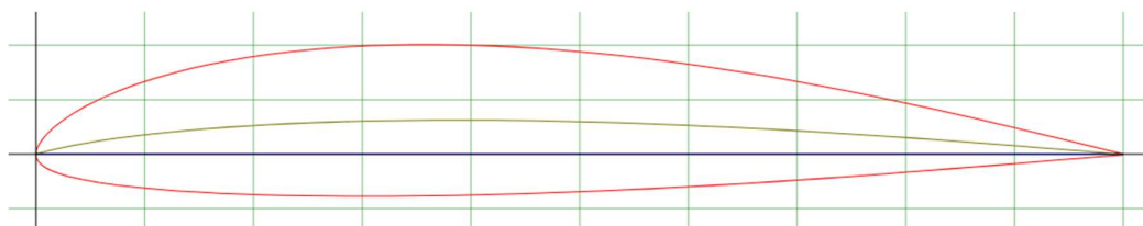
Рис. 3.8. Drela MRC-16
