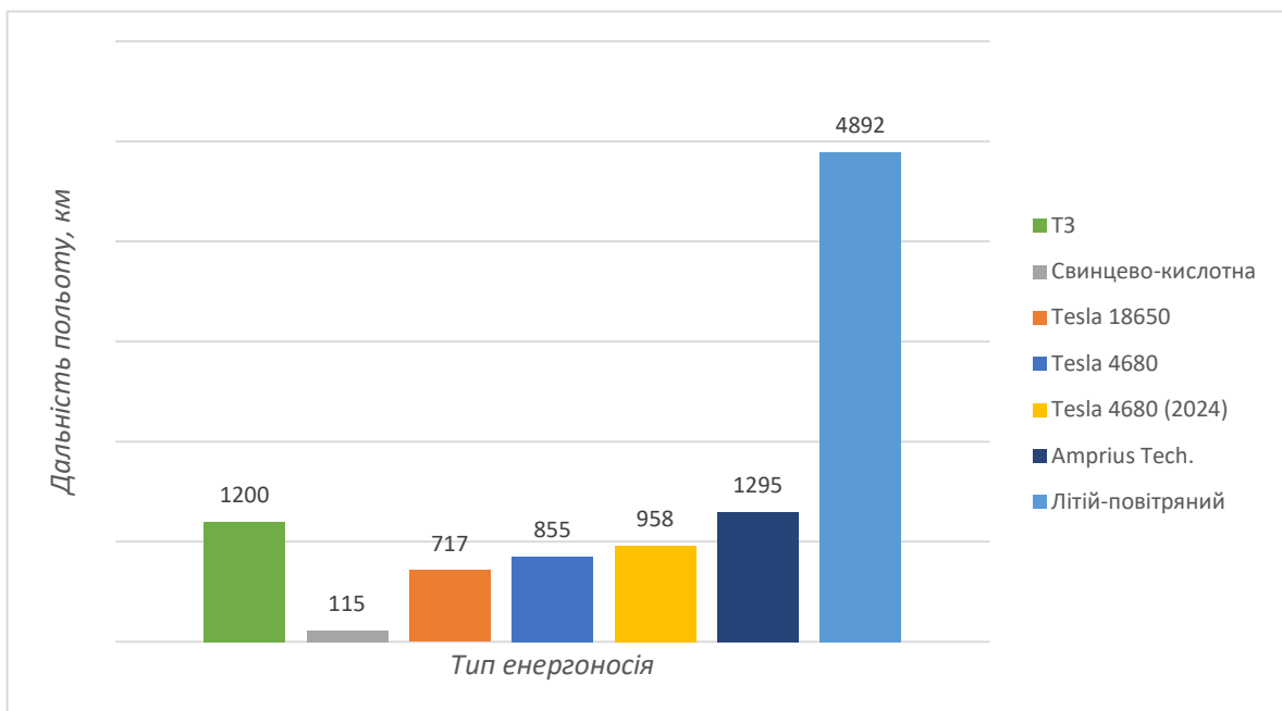
Рис. 5.8. Діаграма порівняння тривалості роботи різних типів енергоносіїв
