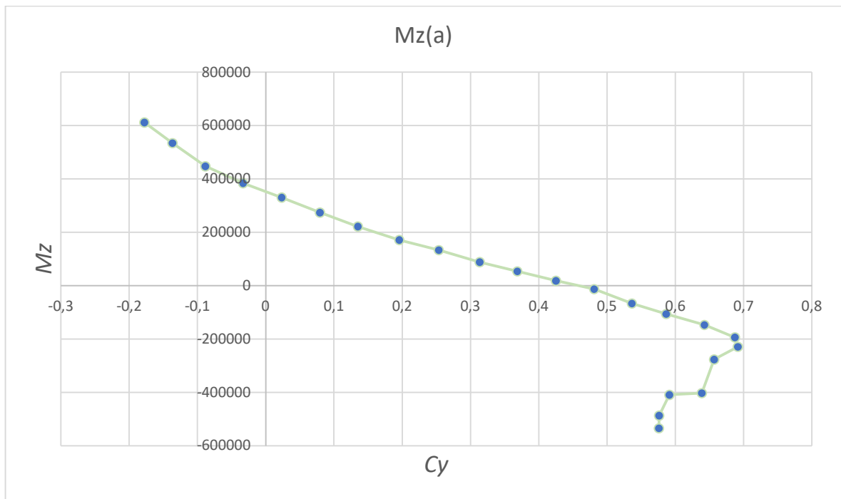
Графік 4.5. Момент навколо поперечної осі відносно коефіцієнта підйомної сили C_y .
