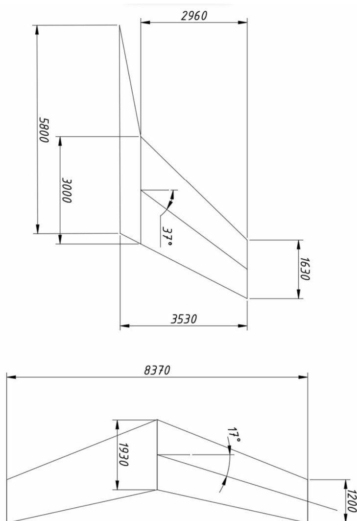
Рис. 3.15. Геометричні характеристики ГО та ВО.
