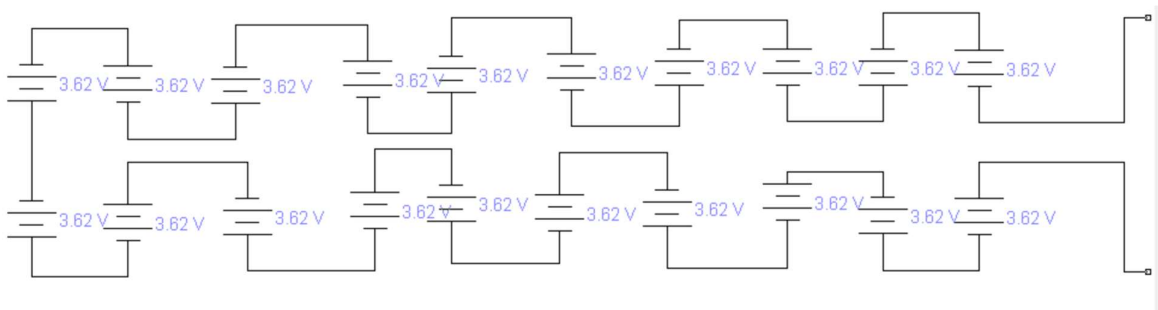
Рис. 7.1. Блок 72V586W
