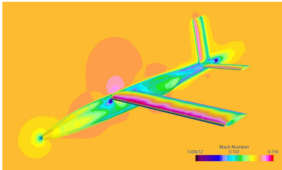
Рис. 4.2 Аеродинамічний розрахунок БПЛА числовими методами.
