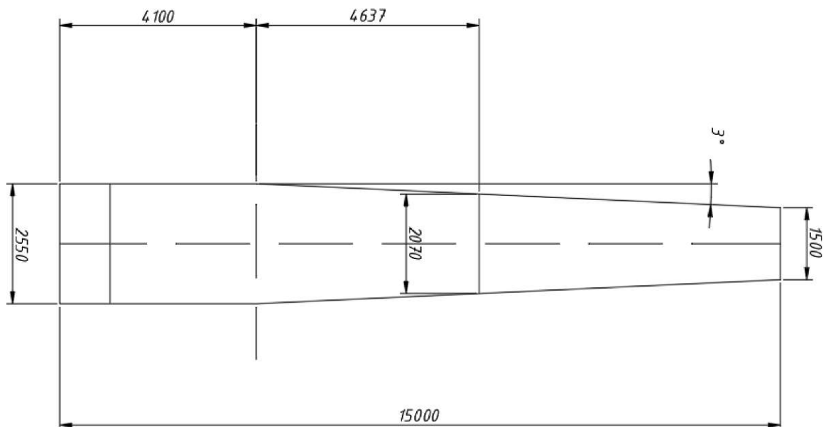
Рис. 3.13. Геометричні характеристики крила.
