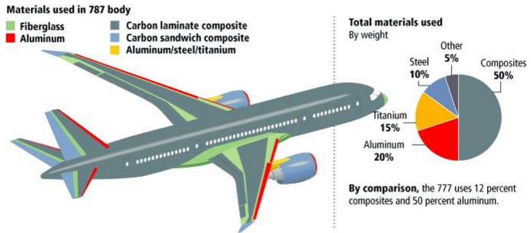
Рис. 6.1. Матеріали використані у Boeing 787 Dreamliner.
