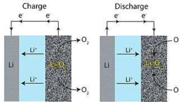
Рис. 5.7. Принцип роботи літій-повітряного акумулятора.
