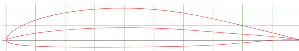
Рис. 3.7. Eppler 434
