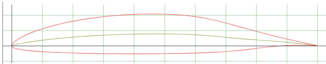
Рис. 3.3. Wortmann 74-130 WP2
