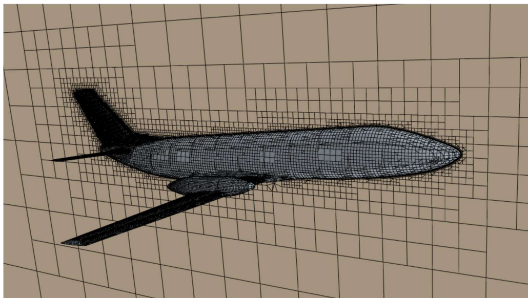
Рис. 4.4. Результат генерації сітки.
