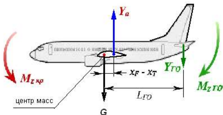
Рис. 3.13. Повздовжня стійкість та керованість літака.
