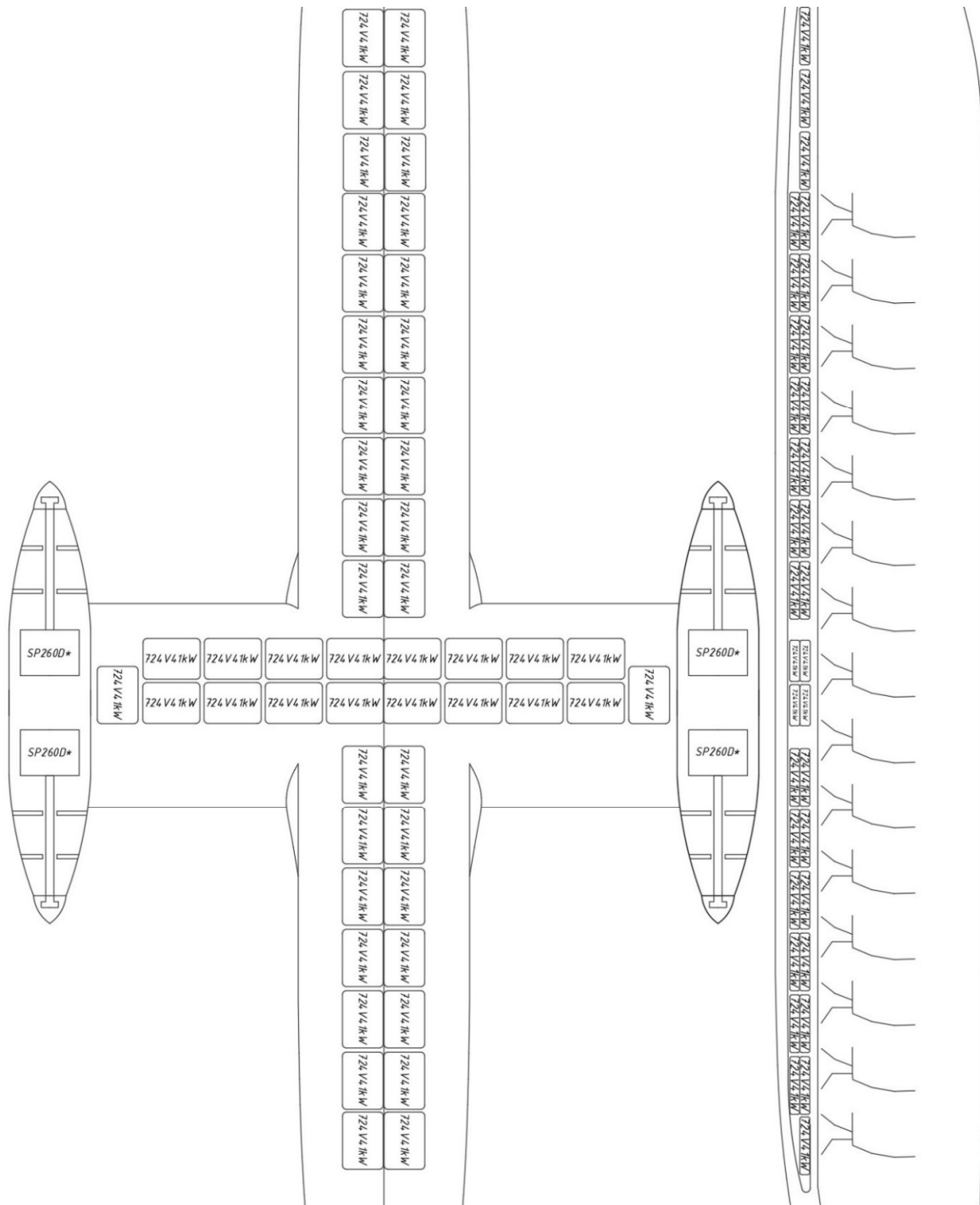
Рис. 7.7. Схема компоновання силової установки та елементів живлення.
