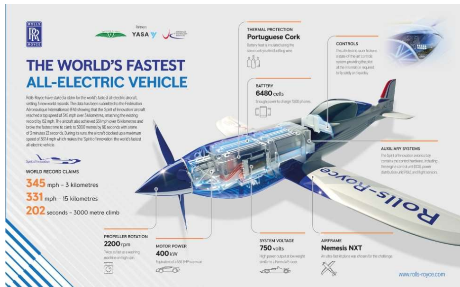
Рис. 1.4. Rolls-Royce's «Spirit of Innovation».
