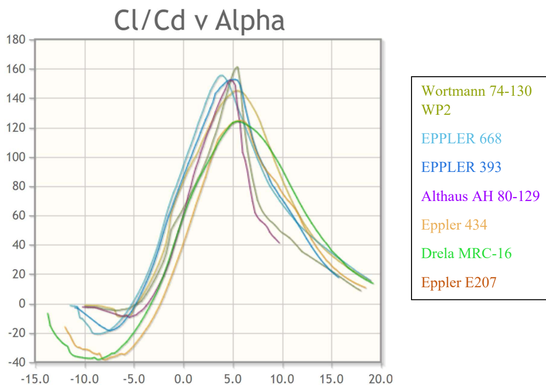
Рис. 3.10. Аеродинамічна якість відносно кута атаки.
