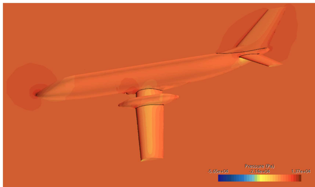
Рис. 4.6. Розподіл тиску при куті атаки -7^\circ .
