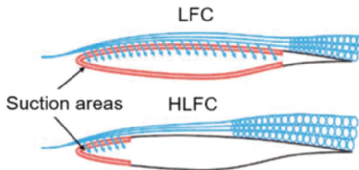
Рис. 6.3. Системи контролю ламінарності потоку.
