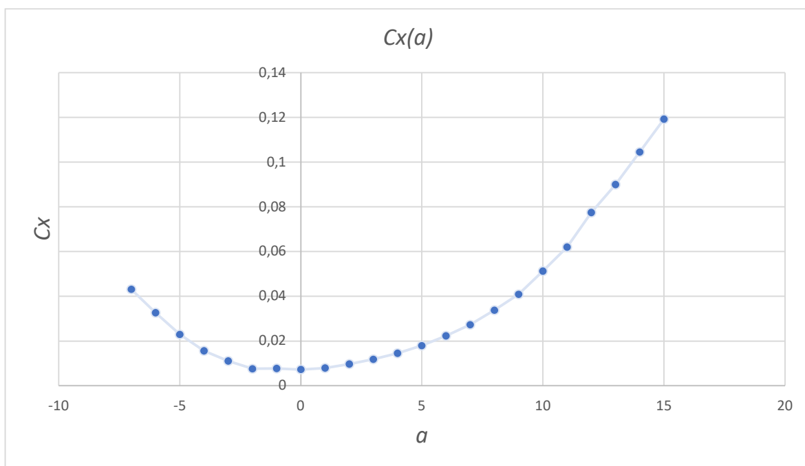
Графік 4.2. Коефіцієнт лобового опору C_x відносно кута атаки \alpha .
