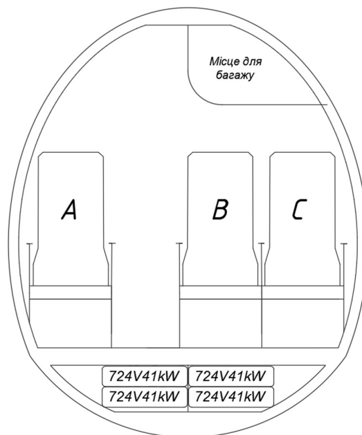
Рис.7.6. Компонування внутрішнього простору фюзеляжу.
