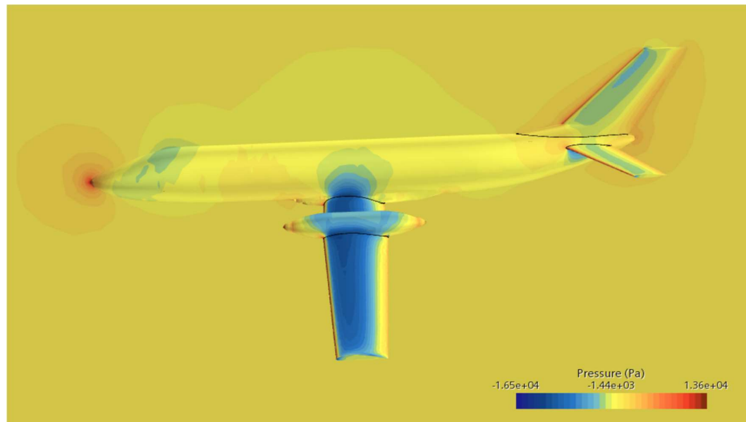
Рис. 4.5. Розподіл тиску при куті атаки 0°.
