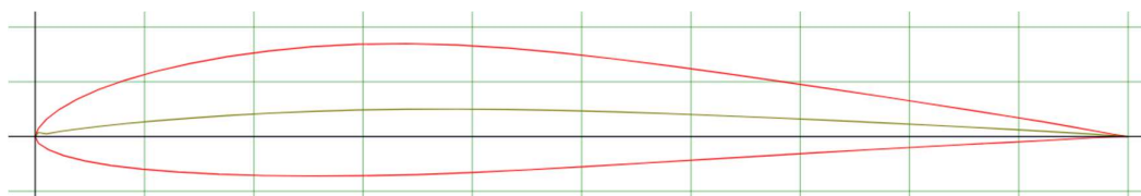
Рис. 3.9. Eppler E207
