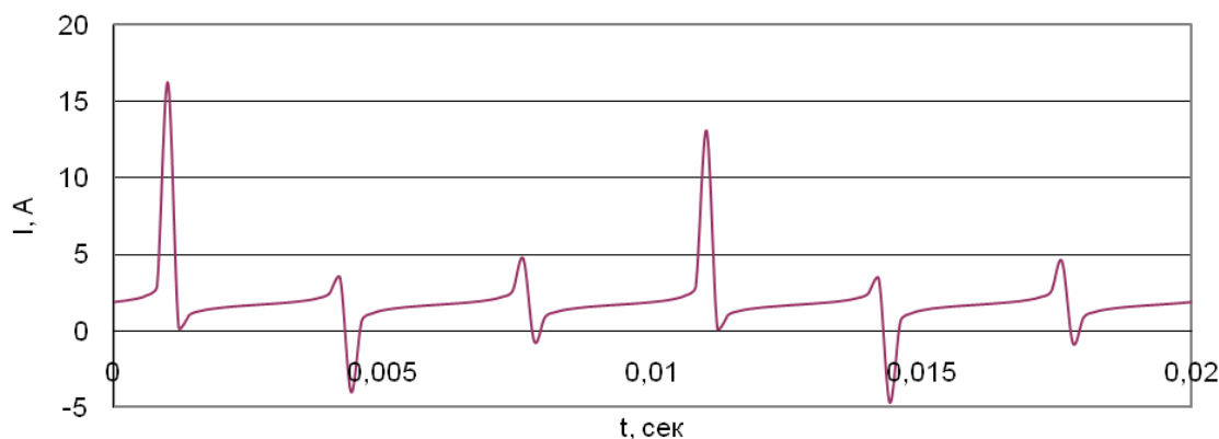
Рис. 1. Відмінність струму, що генерує РП i_{p,PI}(t) , від сумарного струму, який повинен бути скомпенсованим i_{p\Sigma}(t)
