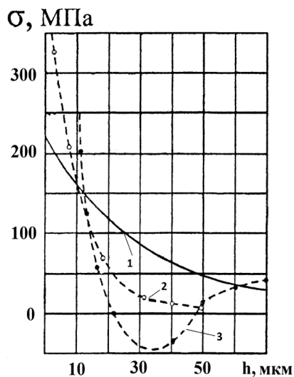
Рис. 1. Вплив зернистості абразивних кругів з карбиду кремнію зеленого (63С) та матеріалу, зв'язки абразиву — керамічної (К), гліфталевої (Гл) на розподіл залишкових напружень поверхневого шару при тонкому шліфуванні композиційного сплаву 86Х6НФТ+5%CaF 2 : 1 — круг 6325СМ2К5; 2 — круг 63С6СМ2Гл; 3 — круг 63СМ14СМ2Гл
