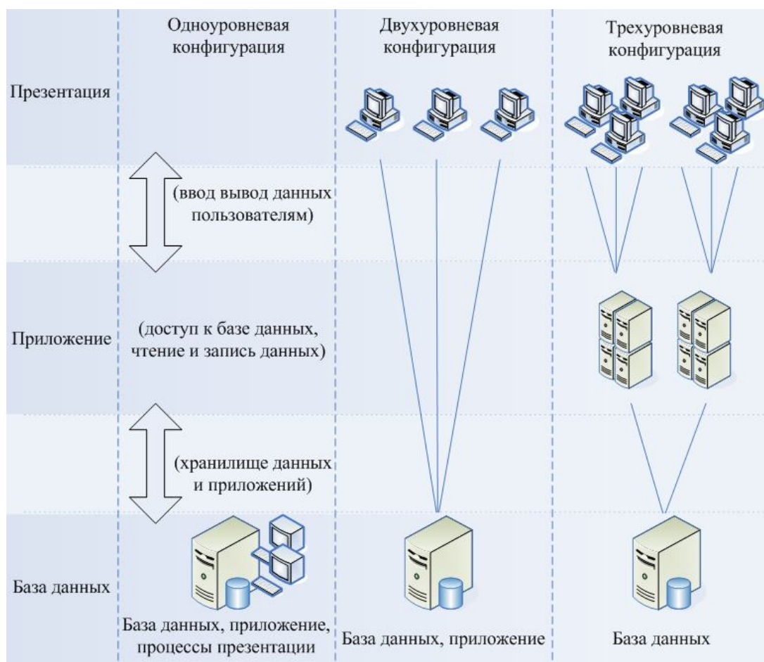
Рисунок 1 – Трёхзвенная архитектура SAP R/3
