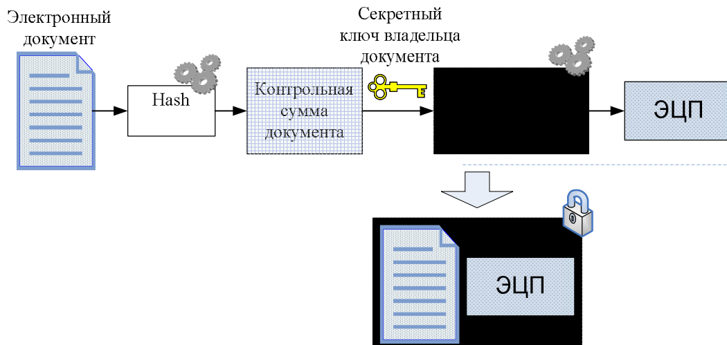
Рисунок 3 – Схема формирования электронной цифровой подписи
