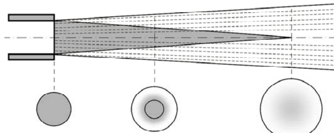
Рис. 2. Виділення ділянок гідралічного струменя
