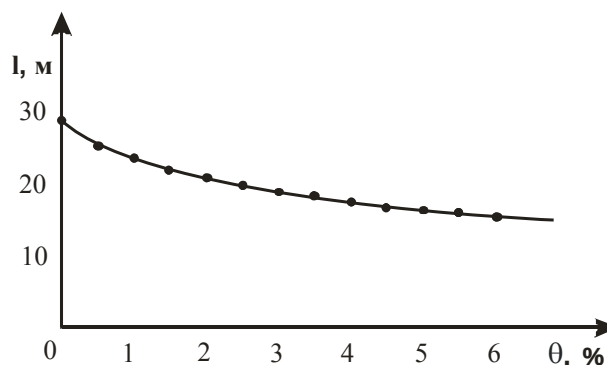
Рис. 4. Максимальна дальність подачі струменя при зміні відсотка розчину піноутворювача
