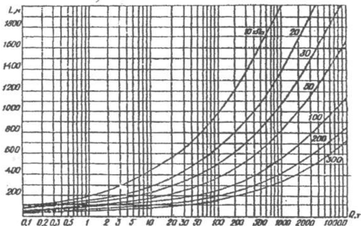
Рис. 12.1. Графіки надмірного тиску в залежності від маси пропану і відстані до центру вибуху
