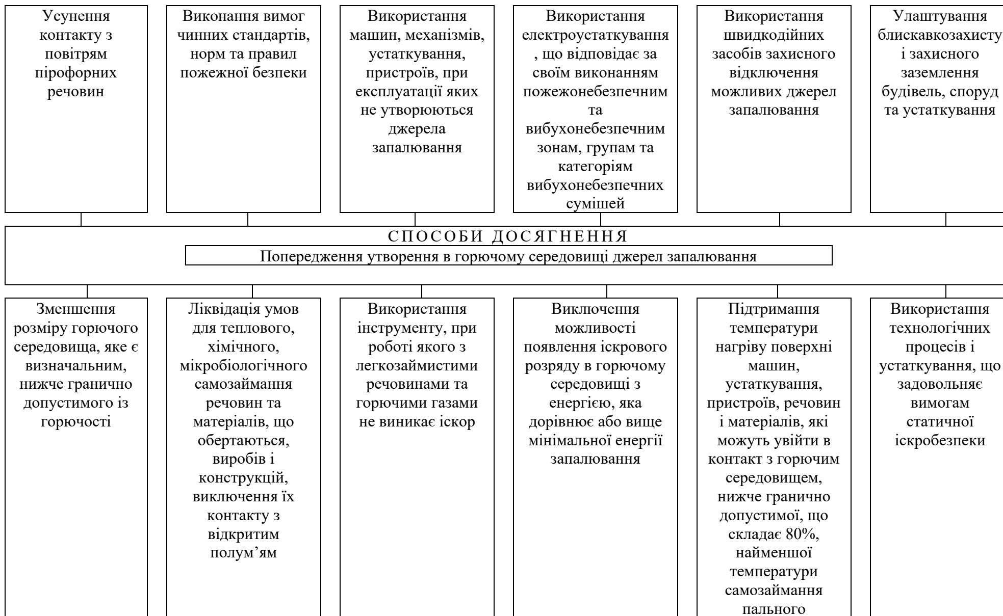
Рис. 11.5 . Схема забезпечення попередження утворення в горючому середовищі джерел запалювання
