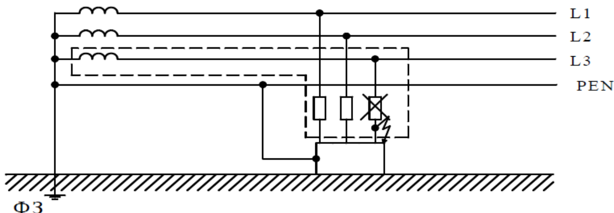
Рис.10.5. Схема захисного заземлення у мережі з глухозаземленою нейтраллю ДЖ напругою до 1 кВ (підсистема TN-C)
