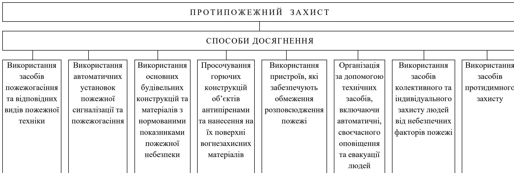
Рис. 11.6 . Схема забезпечення протипожежного захисту
