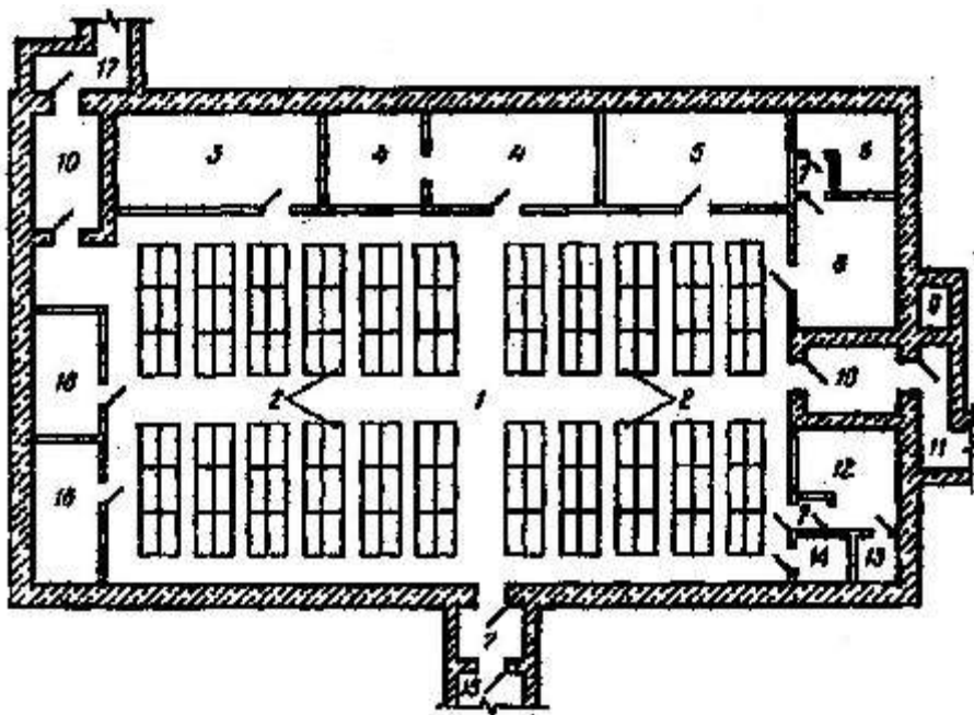
Рис. 13.1. План сховища:
