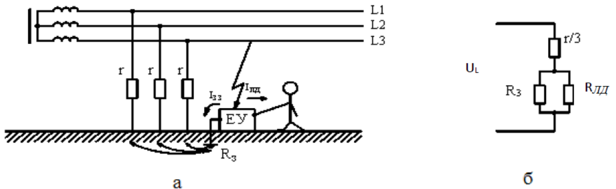
Рис.10.4. Схема захисного заземлення у мережі з ізолюованою нейтраллю ДЖ (система ІТ): а – схема електрична; б – схема еквівалентна; r – опір витoku фазних проводів ЕМ; R_з – опір заземлюючого пристрою; R_{лД} – опір людини; I_{зз} – струм замикання на землю; I_{лД} – струм через людину; U_L – фазна напруга.
