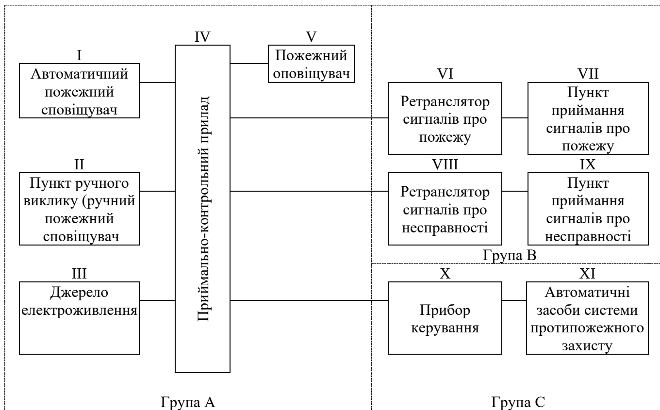
Рис. 11.7. Схема системи пожежної сигналізації
