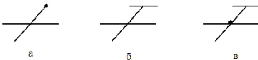
Рис. 10.1. Умовне позначення провідників у системах заземлення: а – N, М – провідників; б – РЕ – провідників; в – PEN – провідників
