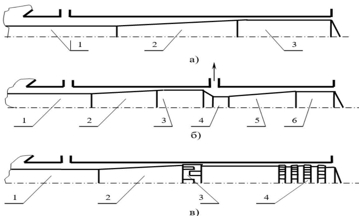
Рисунок 14.21 – Типи односторонніх екструдерів
