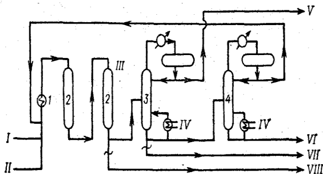
Рисунок 7.6 – Установка одержання МТБЕ
