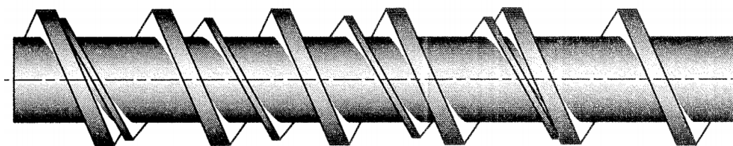
Рисунок 14.7 – Шнек Майллефера
