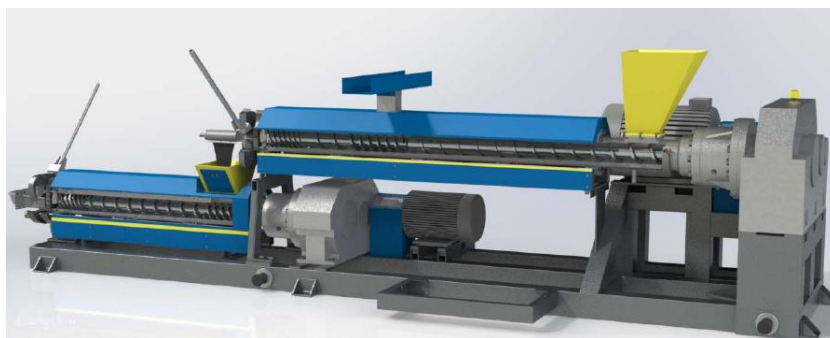
Рисунок 14.16 – Каскадний екструдер SLE-K-125-125
