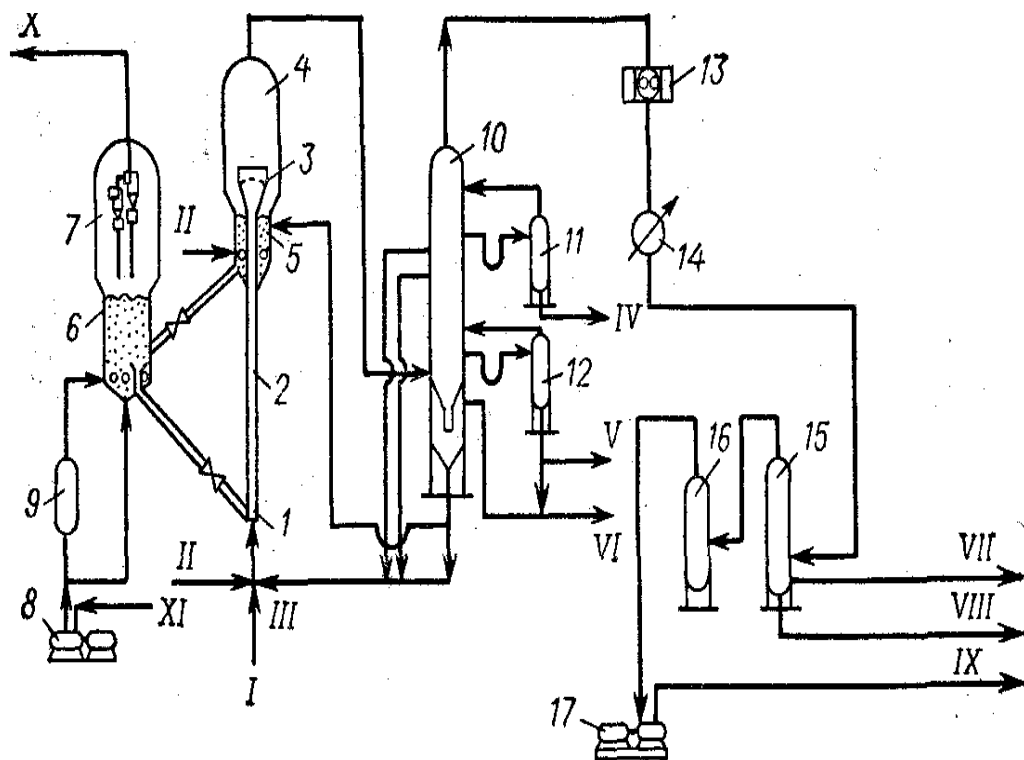
Рисунок 4.1 – Установка термокаталітичного крекінгу
