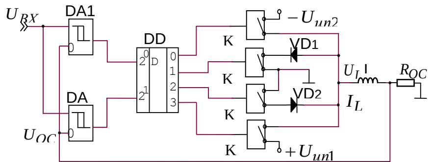
Рис. 6. Підсилювач струму індукторів
