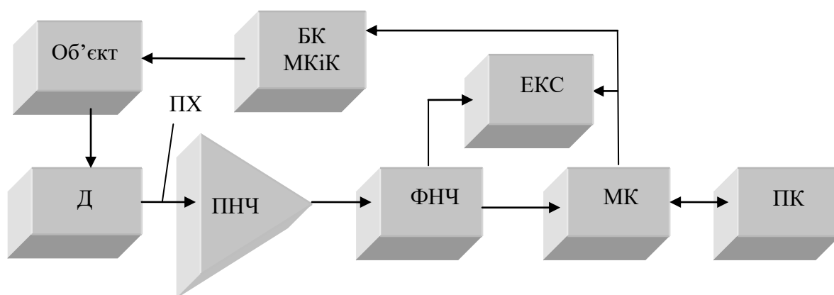
Рис. 2. Підсистема програмно-апаратної обробки сигналу ПХ: Д – тензодатчик, МК – мікроконтролер, ПНЧ – підсилювач низької частоти, ФНЧ – фільтр нижніх частот, ЕКС – екстрематор, БК МКіК – блок керування мікроконтролером і клапаном, ПК – персональний комп'ютер
