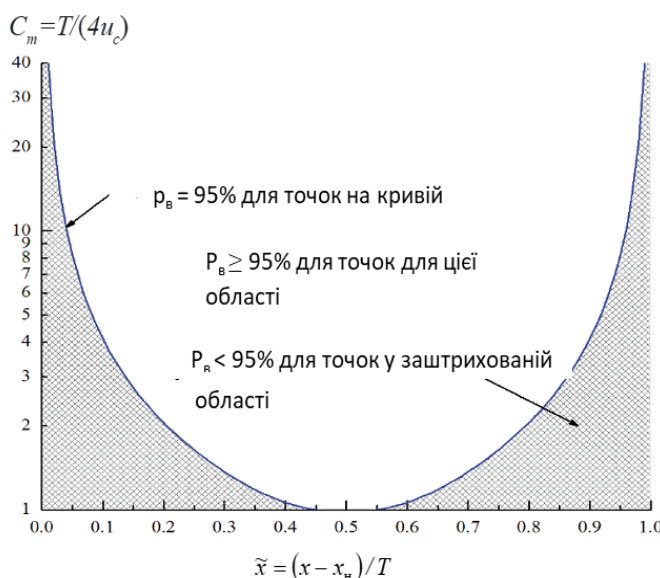
Рисунок 6 – Взаємозв'язок C_m, p_v та \tilde{x}
