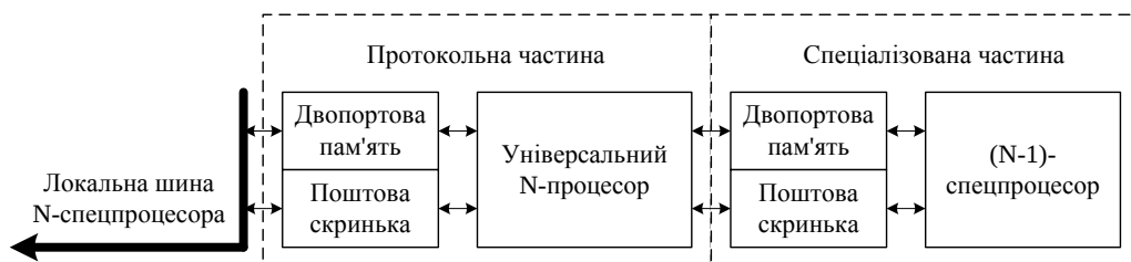
Рисунок 3 – Структура N-спецпроцесора
