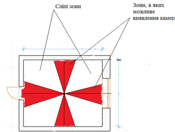
Рис. 5. Діаграма спрямованості лазера та приймального пристрою
