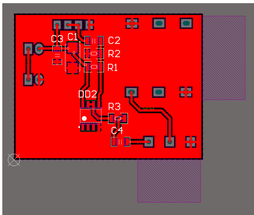
Рисунок 3.13 — Трасування ДП
