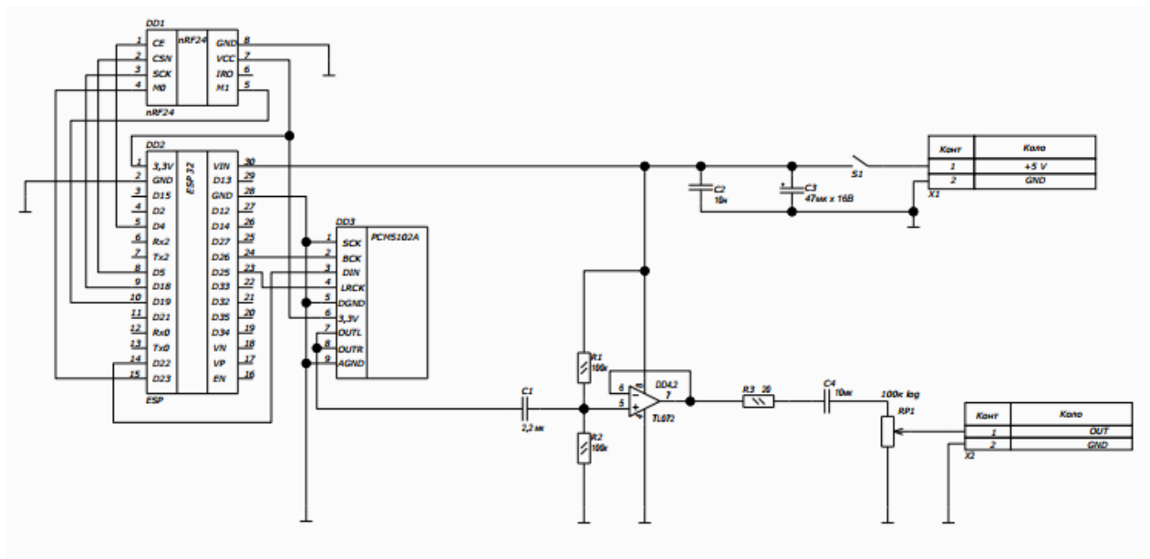
Рисунок 2.10 — Схема приймача на основі модуля nRF24
