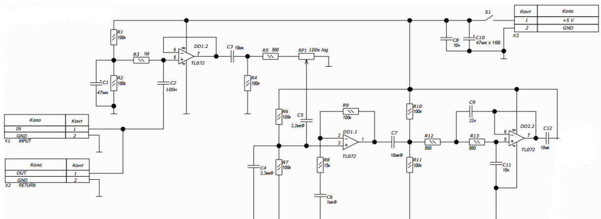
Рисунок 2.1 — Вдосконалена схема аналогової частини передавача.
