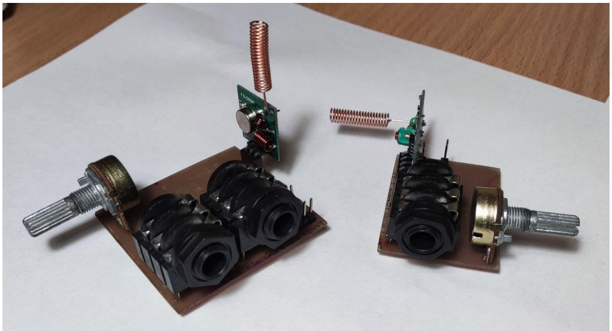
Рисунок 3.19 — АМ прототип
