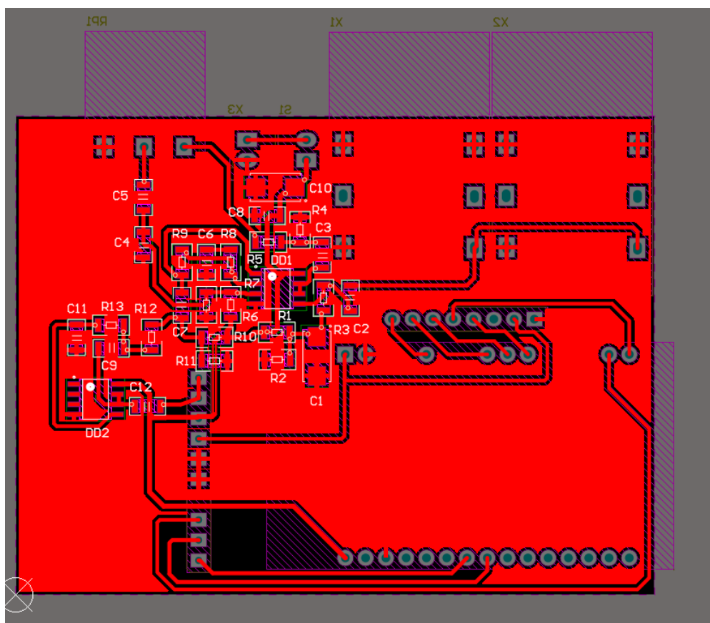
Рисунок 3.11 — Трасування ДП
