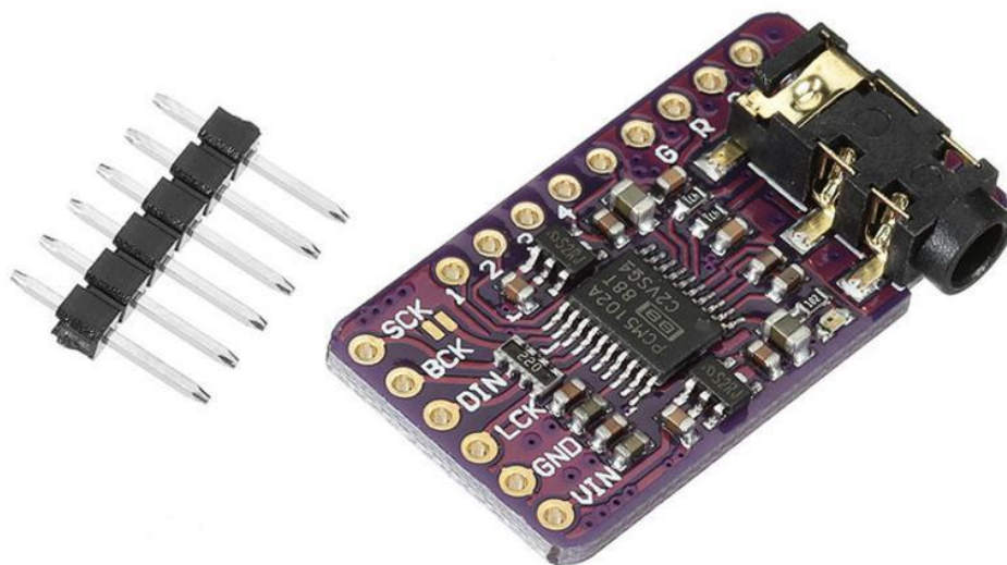
Рисунок 3.2 — Модуль ЦАП PCM5102A
