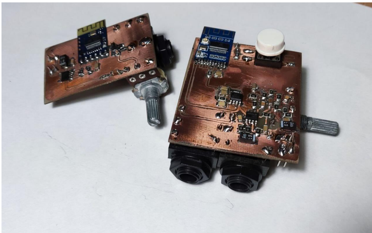
Рисунок 3.20 — Bluetooth прототип
