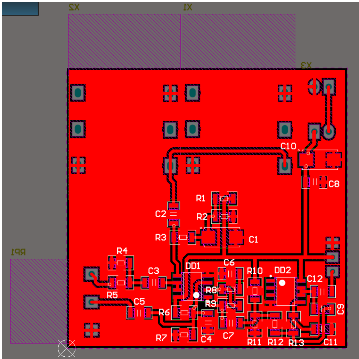
Рисунок 3.6 — Трасування ДП
