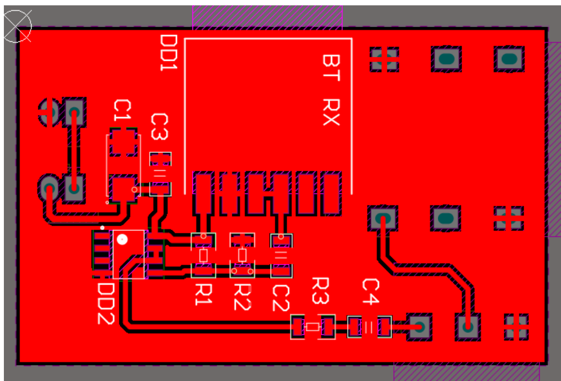
Рисунок 3.15 — Трасування ДП
