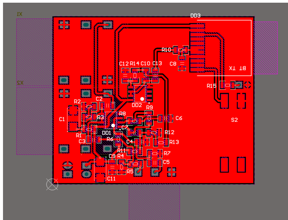
Рисунок 3.8 — Трасування ДП
