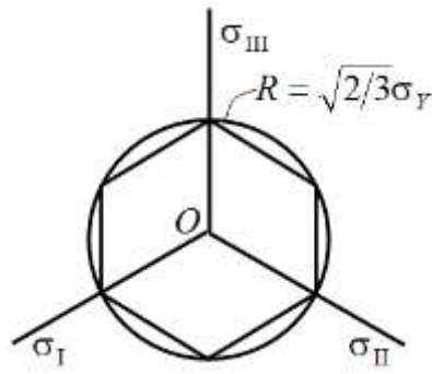
Рис. 8.4. Коло Мізеса
