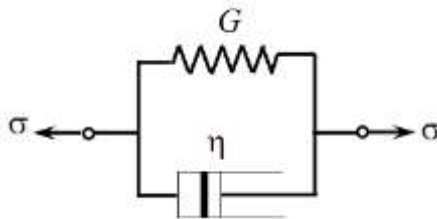
Рис. 9.2. Модель в'язко-пружного середовища Кельвіна
