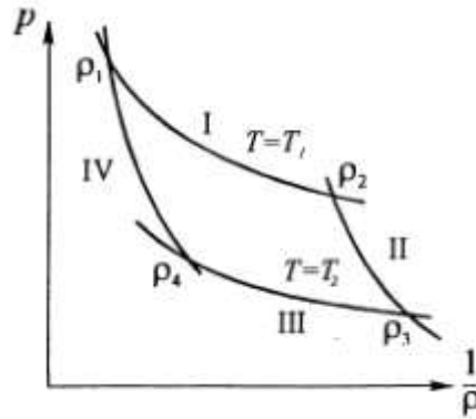
Рис. 7.6. p - v діаграма циклу Карно
