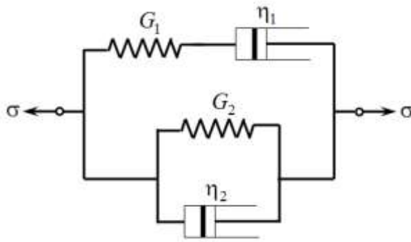
Рис. 9.19. Комбінована модель Кельвіна-Максвела
