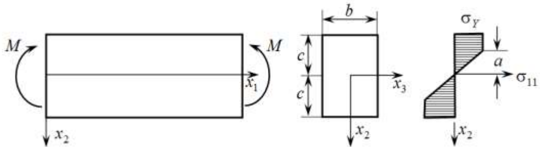
Рис. 8.6. Згин балки
