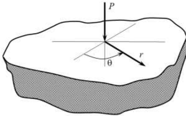
Рис. 9.17. Напівпростір із в'язко-пружного матеріалу Кельвіна, до якого прикладене концентроване навантаження P
