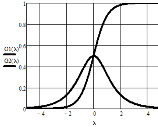
Рис. 9.22. Графіки функцій G_1(\lambda) = \frac{Ge^{2\lambda}}{1+e^{2\lambda}} і G_2(\lambda) = \frac{Ge^{\lambda}}{1+e^{2\lambda}} за умови G=1
