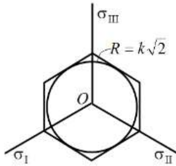
Рис. 8.16. Криві текучості, що відповідають критерию Треска
