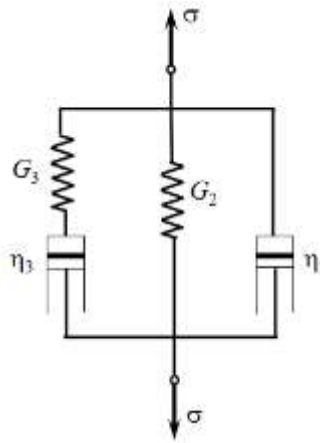
Рис. 9.6. Вироджений випадок узагальненої моделі Максвела
