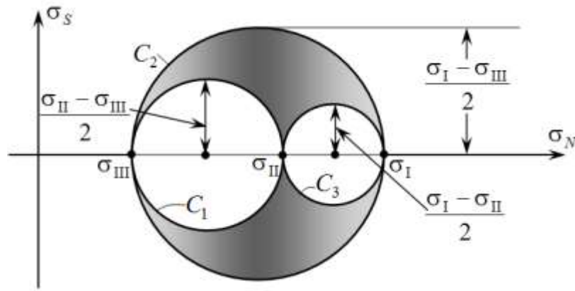
Рис. А.2. Круги Мора
