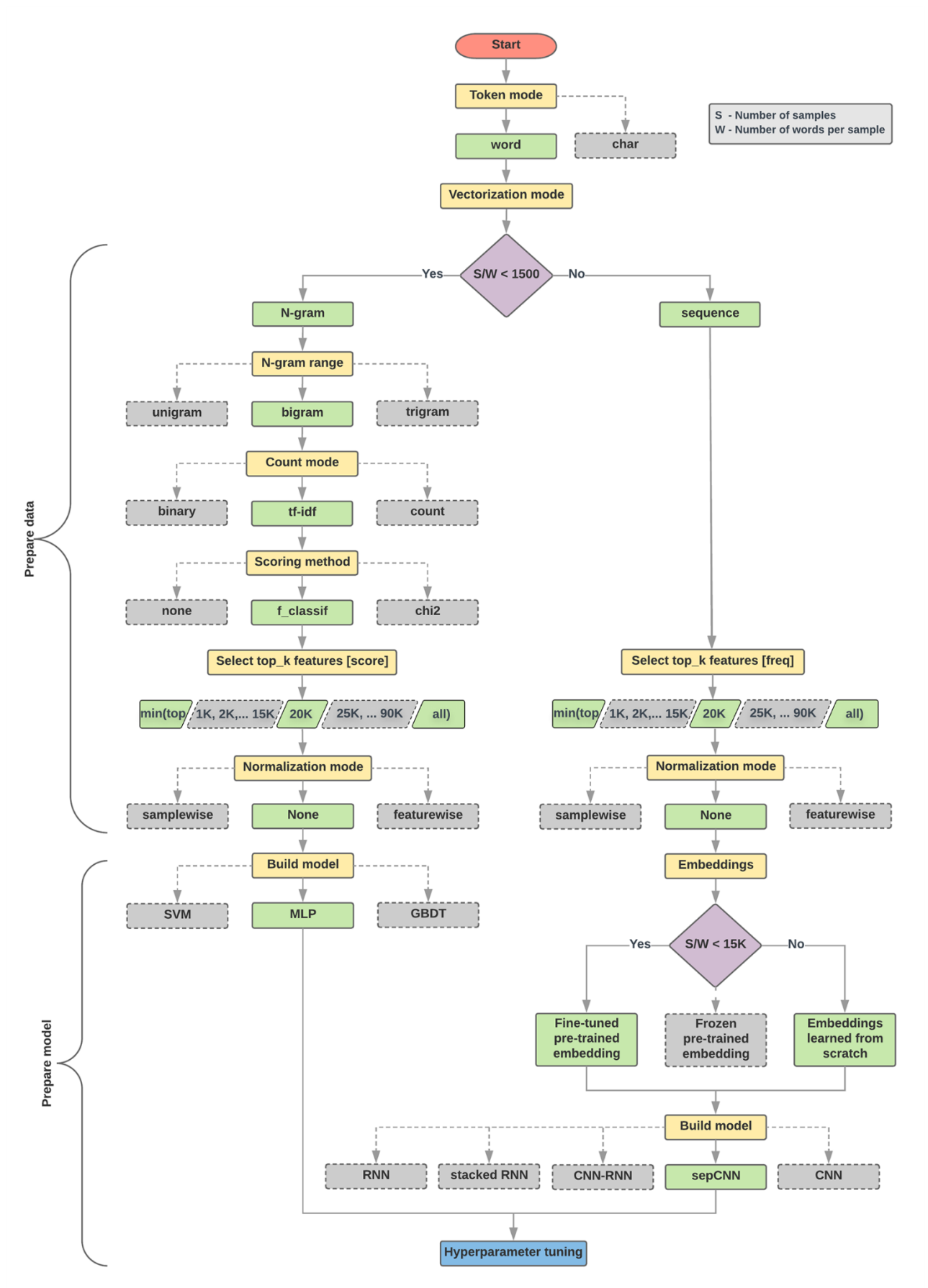
Рисунок 1.14 - Блок-схема вибору моделі класифікації тексту
