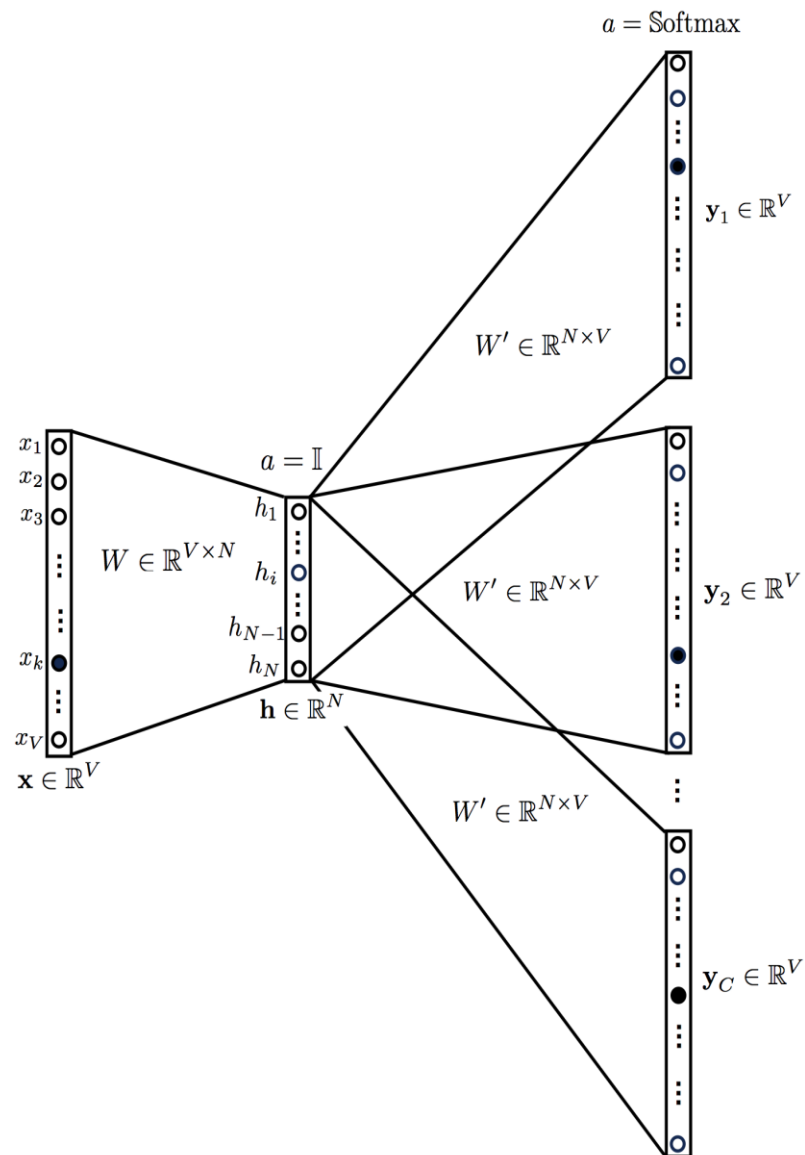
Рисунок 1.10 - Архітектура моделі Skim Gram
