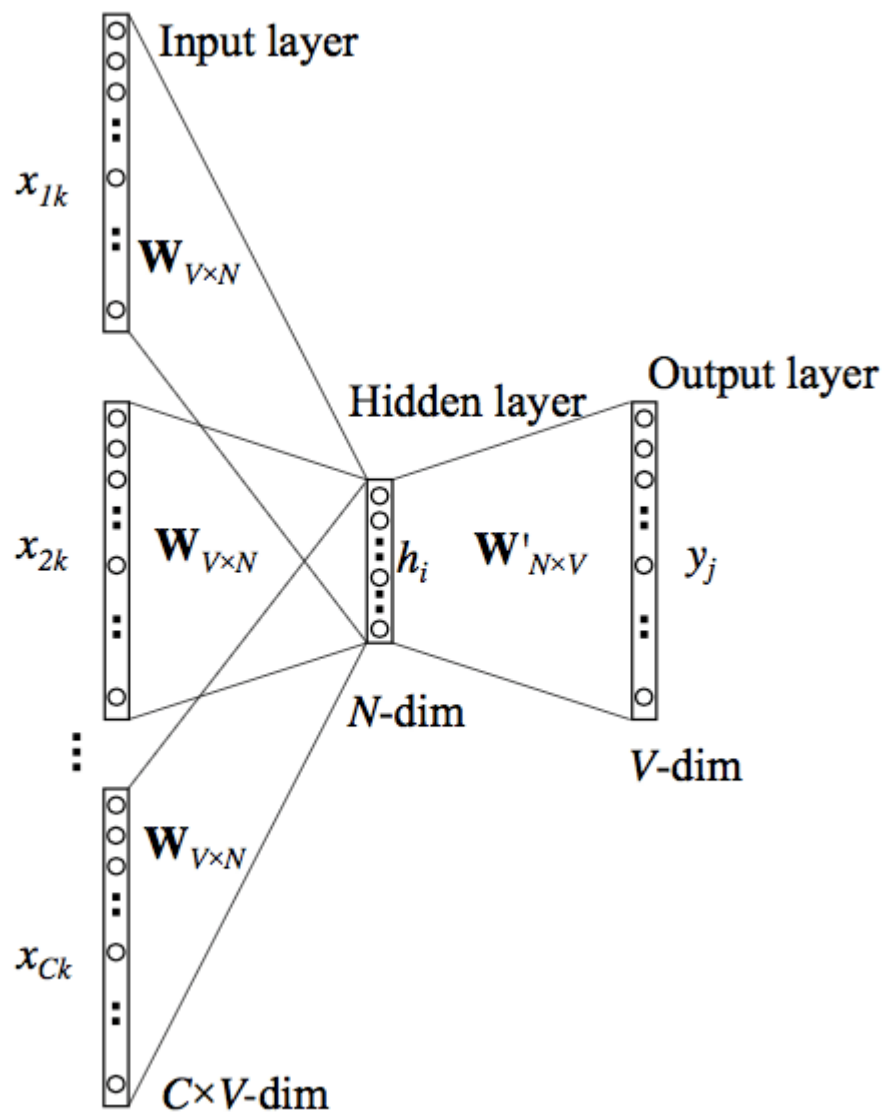
Рисунок 1.9 - Модель CBOW з кількома словами контексту
