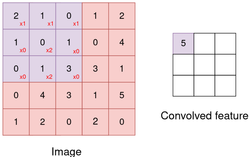
Рисунок 1.17 - Операція згортки
