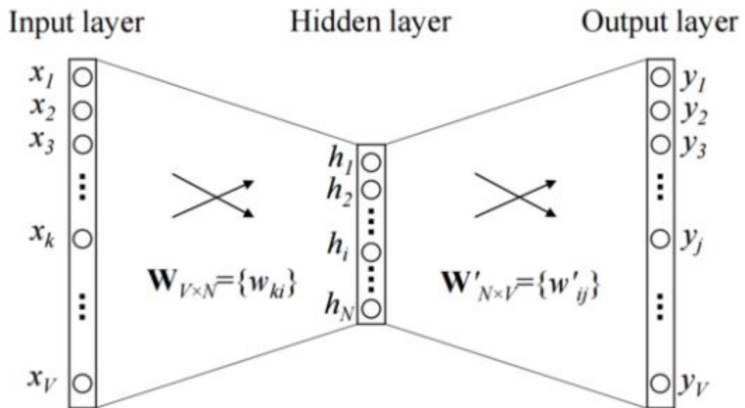
Рисунок 1.8 - Проста модель CBOW з одним словом контексту
