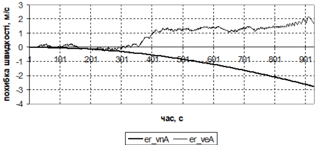
Рис. 18. Похибка північної та східної швидкості в автономному каналі
