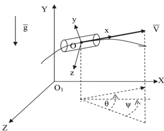
Рис. 8. Топоцентрична і зв'язана системи координат
