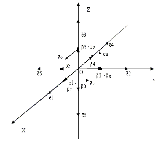
Рис. 3 Схема розміщення дев'яти АК в блоці
