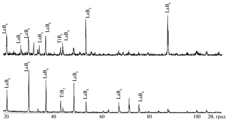
Рис. 5. Дифрактограма сплаву \text{LaB}_6\text{-TiB}_2 + 1\% (за масою) В, отриманого шляхом розпилення на мідну пластинку (а) і відцентровим розпиленням (б).
