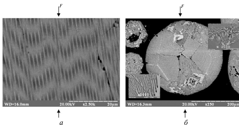
Рис. 7. Мікроструктура зразків системи \text{LaB}_6\text{-TiB}_2 : спрямовано закристалізований стрижень (а) і армований полікристалічний порошок, отриманий за методом відцентрового розпилення (б).
