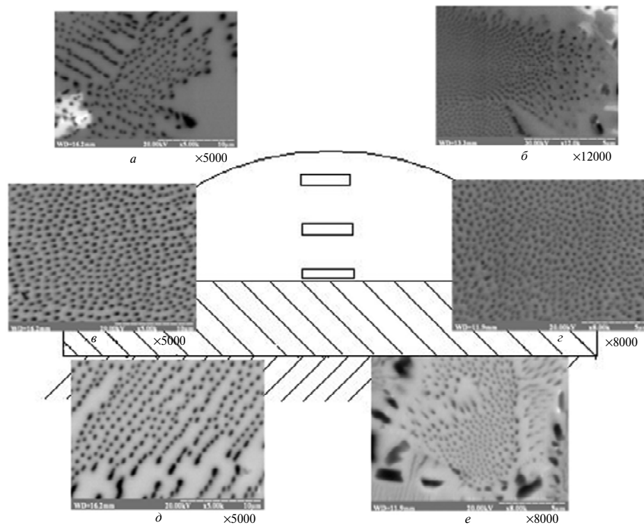
Рис. 4. Мікструктура крапель розплаву евтектичного сплаву систем \text{LaB}_6\text{-TiB}_2 + 1\% (за масою) (а, в, г) і \text{LaB}_6\text{-TiB}_2 + 2\% (за масою) В (б, г, е), закристалізованих на мідній пластині: верх (а, б), середина (в, г) і низ (г, е) краплі.
