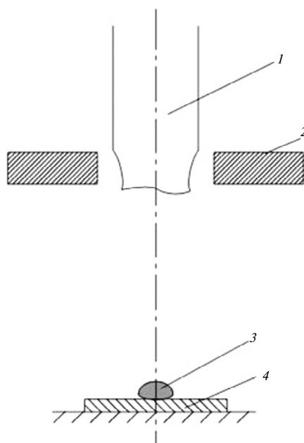
Рис. 1. Схема отримання краплі методом оплавлення стрижня евтектичного сплаву системи \text{LaB}_6\text{-TiB}_2 , вирощеного методом безтигельної зонної плавки: 1 – стрижень; 2 – індуктор; 3 – крапля; 4 – мідна підкладка.
