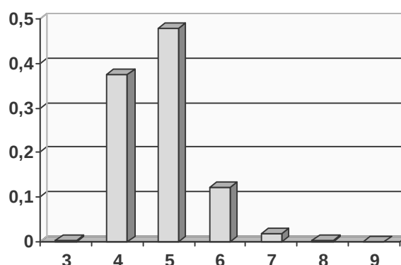
Рисунок 2 – Ймовірність значення параметра t для 8 \times 8 S -блоків.
