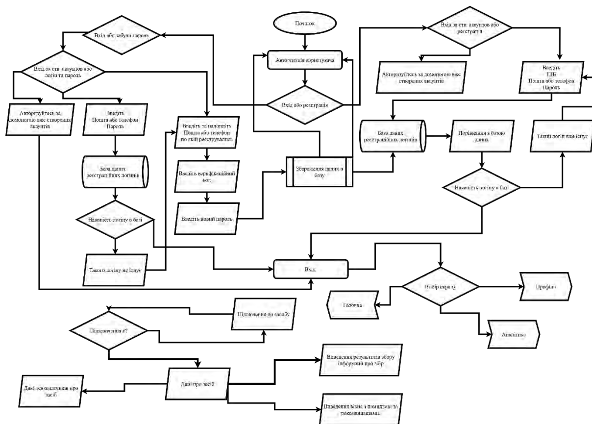
Рисунок 3.2 — Алгоритм роботи мобільного застосунку
