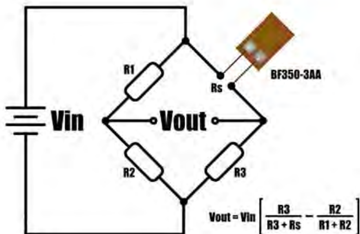
Рисунок 2.4.2 — Мостова схема підключення тензорезисторів
