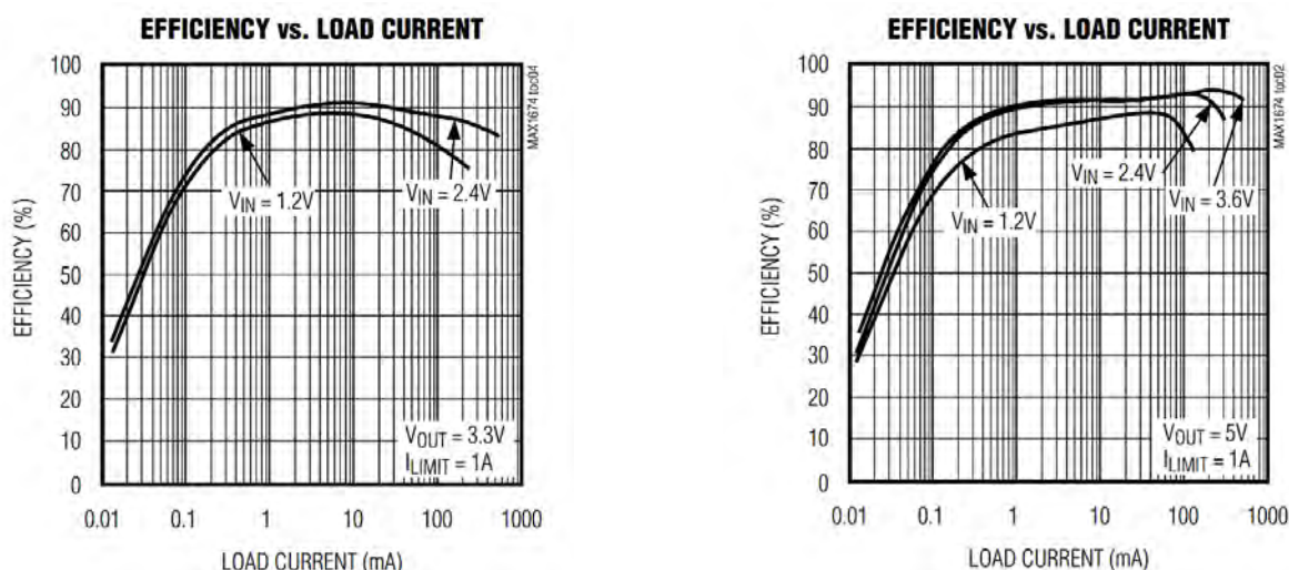
Рисунок 2.3.5 — Ефективність проти струму навантаження при вихідних напругах 3.3 та 5 В
