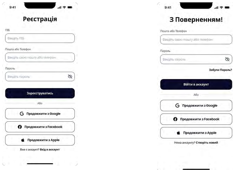
Рисунок 3.3.2 — Авторизація користувача
