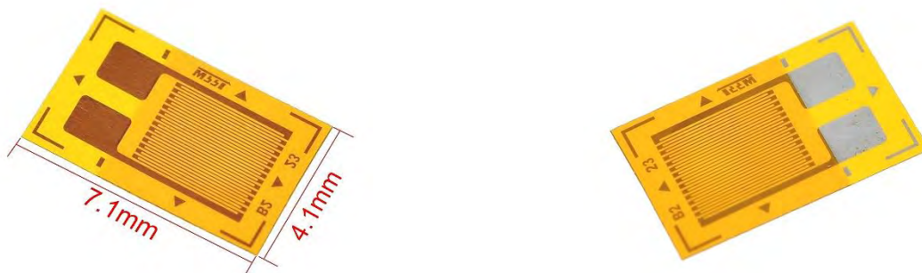
Рисунок 2.3.2 — Плівкового тензорезистор BF350-3AA
