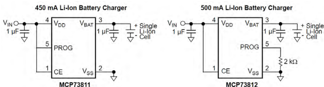
Рисунок 2.2.17 — Типове застосування для зарядки акумулятора варіантом MCP73812
