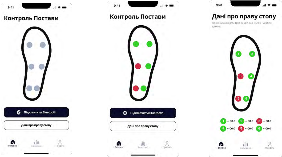
Рисунок 3.3.4 — Головний екран для правої стопи
