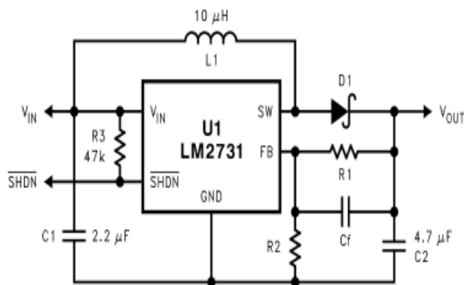
Рисунок 2.2.20 — Типове застосування для стабілізації напруги варіантом LM2731
