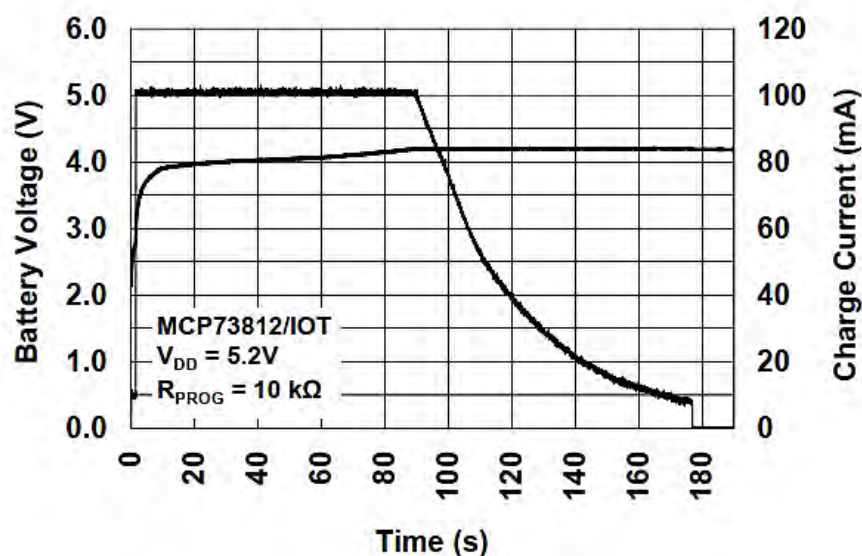
Рисунок 2.3.4 — Типовий профіль заряду (приклад на акумуляторі 180 мА/год)
