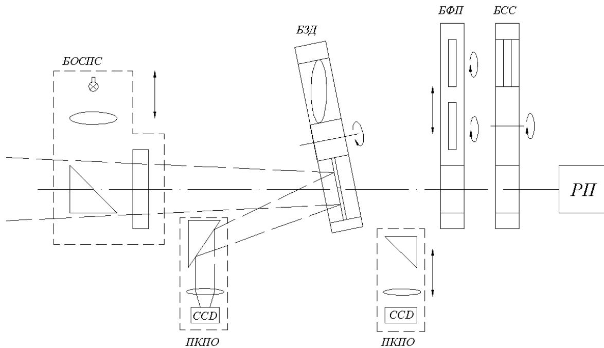
Рисунок 1 – Схема реалізації уніфікованого оптико-механічного блоку. БОСПС – блок опорного спектро-поляриметричного стандарту, БЗД – блок змінних діафрагм, БФП – блок фазових пластинок, РКПО – пристрій контролю положення об'єкта, БСС – блок спектральної селекції, РП – реєструючий пристрій.
