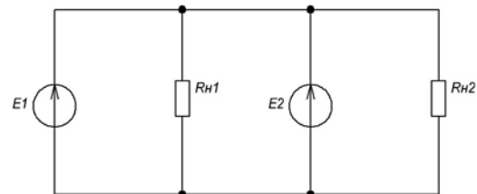
Рис. 4. Сеть с двумя источниками
