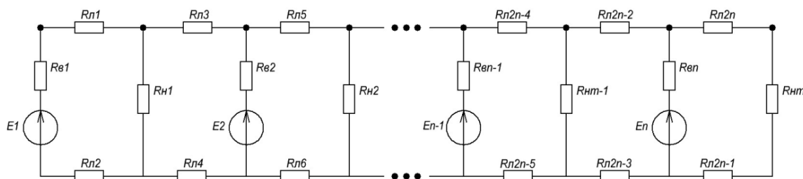
Рис. 1. Электрическая схема, соответствующая сети Смарт Грид
