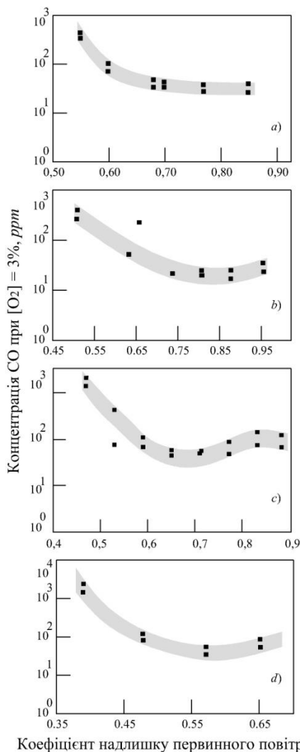
Рис 1. Залежність концентрації CO від коефіцієнту надлишку первинного повітря. Паливо – природний газ. Пальник побутової газової плити «WHIRLPOOL», досліди а – 500, б – 1000, в – 1500, д – 2500.
