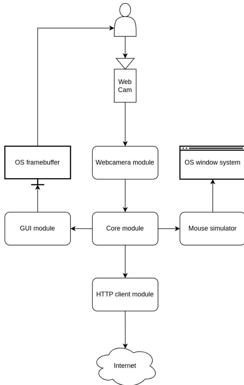
Рисунок 3.3 – Архітектура клієнту
