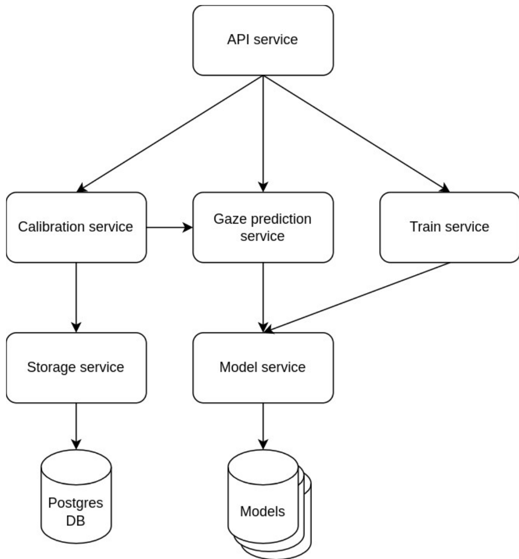
Рисунок 3.2 – Архітектура сервера
