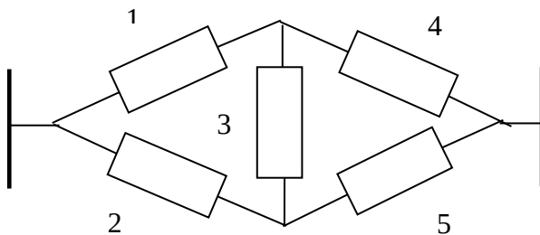
Рис. 1. Структурно-логічна схема до визначення рівня надійності
