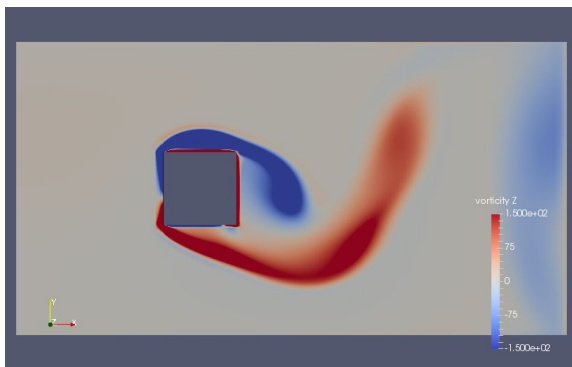
Рис 4.4 Миттєві поля поперечної компоненти завихреності \omega_z
