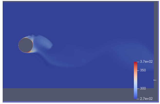
Рис. 4.3 Поле температури при Re = 8 \cdot 10^3
