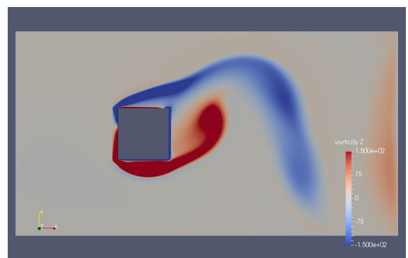
Рис 4.4 Миттєві поля поперечної компоненти завихреності \omega_z
