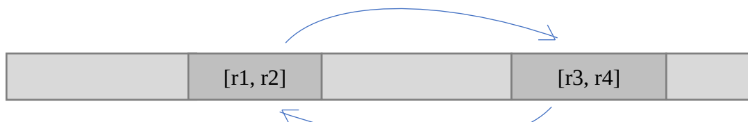
Рисунок 2.3. Мутація хромосом
