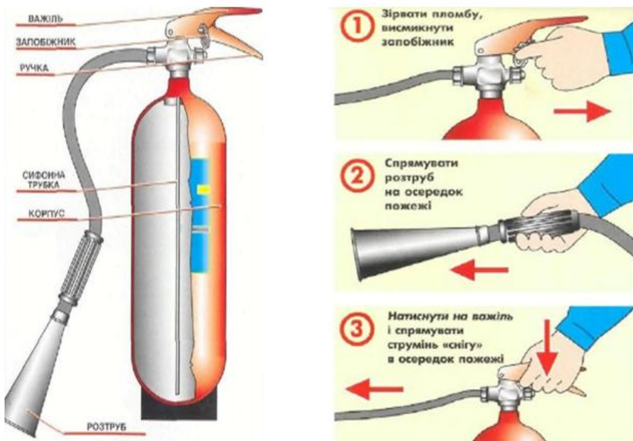
Рис. 14.6. Будова та спосіб приведення в дію вуглекислотного вогнегасника
