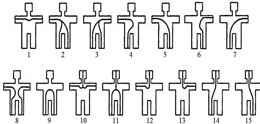
Рис. 17.1. Шляхи проходження струму крізь тіло людини:
