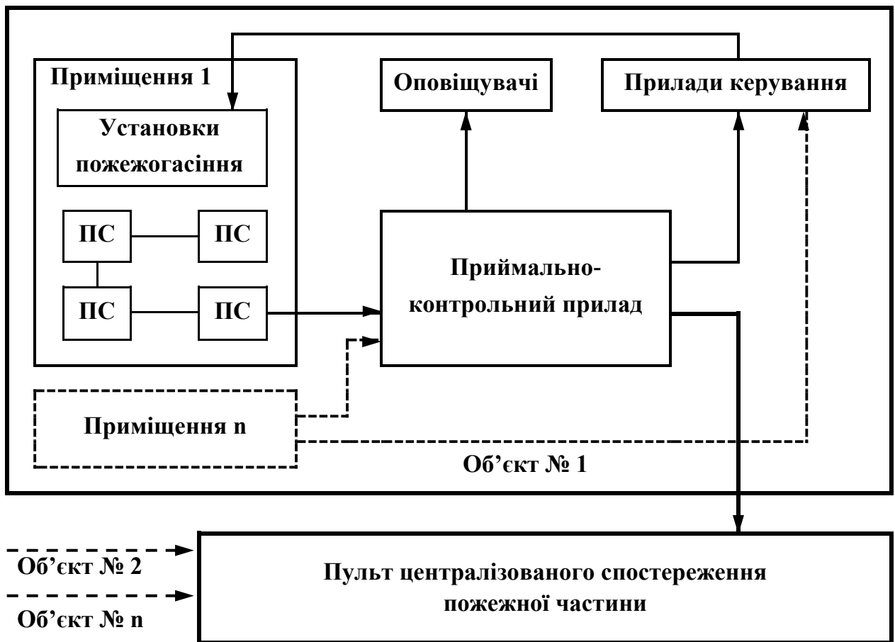
Рис. 14.2. Схема системи пожежної сигналізації (ПС – пожежний сповіщувач)
