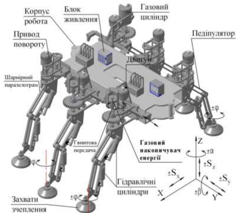
Рис. 3.3. Мобільний робот з пневматичним накопичувачем енергії
