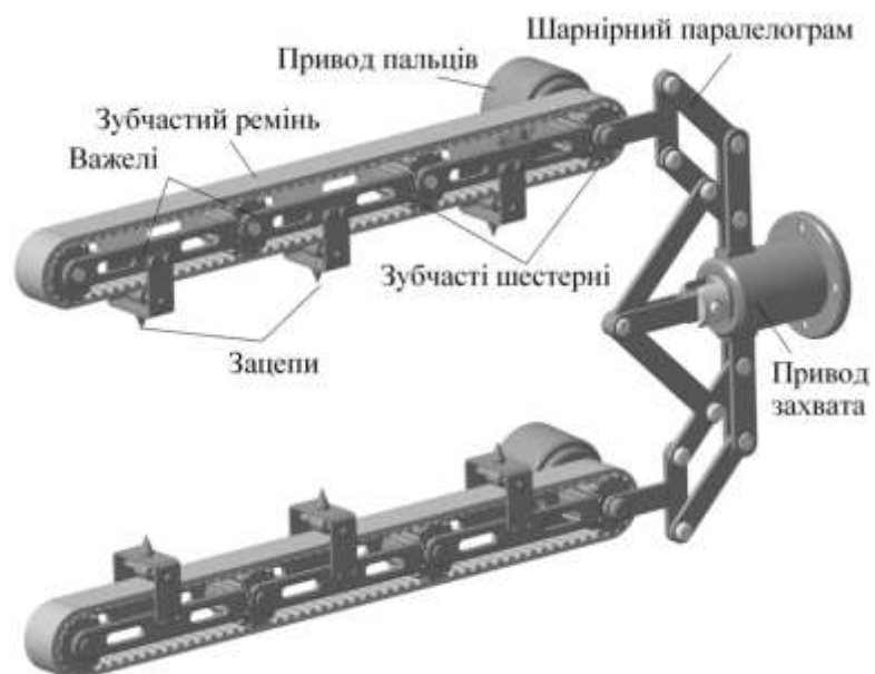
Рис. 15-Л. 3D модель захвата
