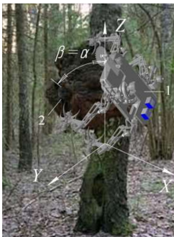
Рис. 4-В. Положення мобільного робота при обрізці наросту 1– робот; 2 – нарост на дереві
