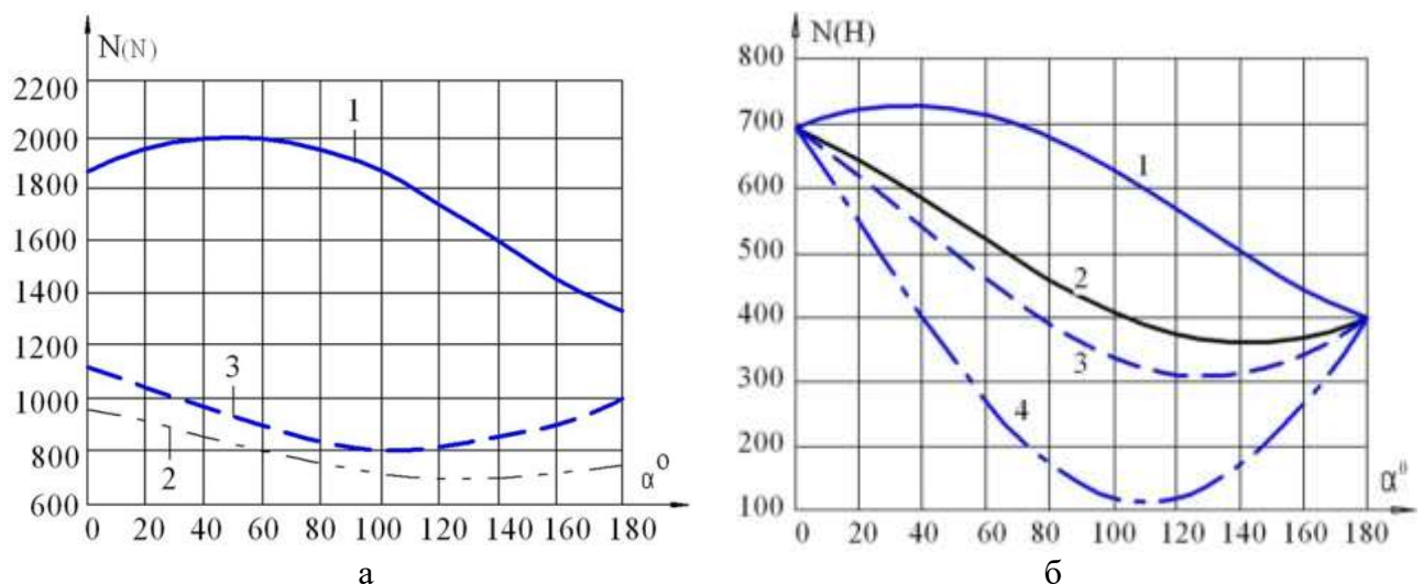
Рис. 4.17. Залежності технологічного навантаження від кута нахилу поверхні переміщення робота при різниці нахилу поверхонь \varphi - \alpha = 30^\circ і коефіцієнті тертя \mu = 0,5 (а) та спираючись на дві ноги (б)
