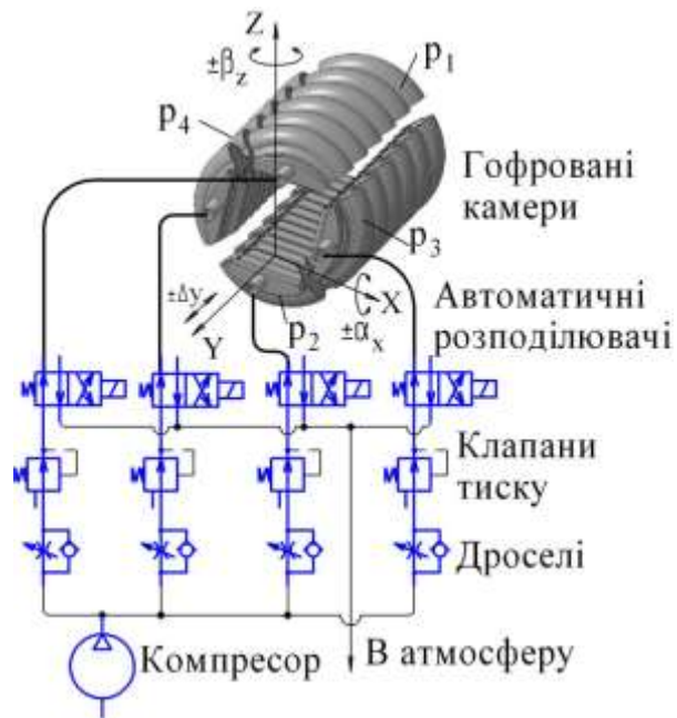
Рис. 4.33. Принципова схема блоку керування гофрованими камерами (м'язами) педипуляторів робота
