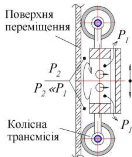
Рис. 1.14. Висхідний транспортний робот з турбогенератором вакууму
