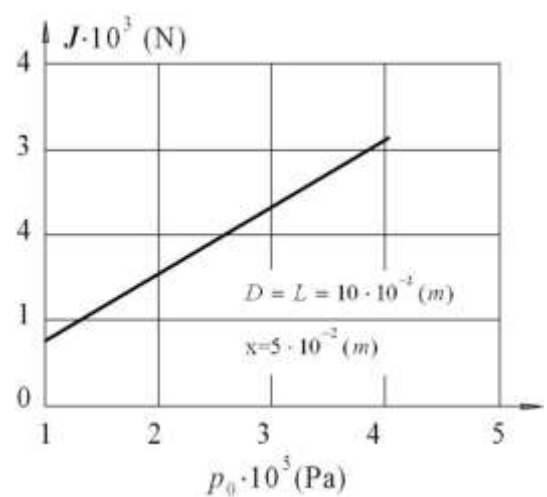
Рис. 3.19. Залежність пружної сили J при зміні початкового тиску в камері
