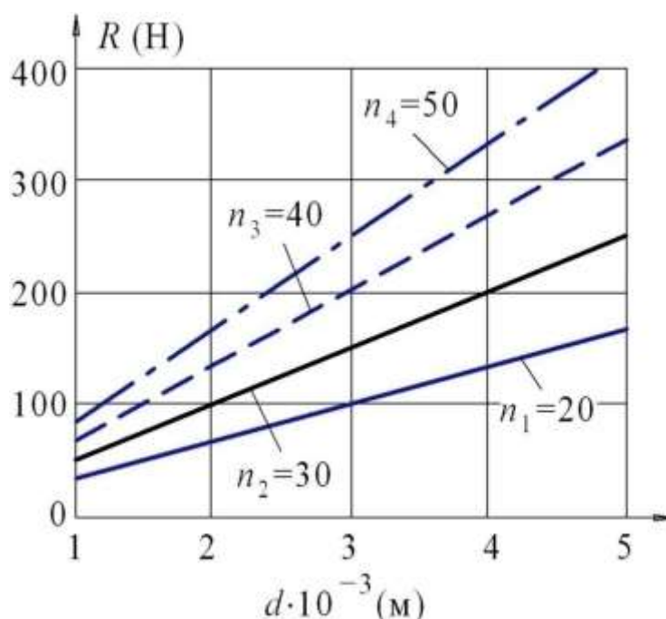
Рис. 6.4. Залежність сили тяги R від діаметрів d отворів і кількості n сопел n при сталому тиску ( p = 6 бар)
