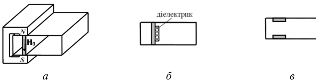
Рисунок 3.7 — Конструкція резонансного вентилля (а) і можливе розташування феритових пластин уздовж вузької (б) та широкої (в) стінки
