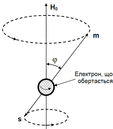
Рисунок 3.2 — Прецесія магнітного моменту електрона у постійному магнітному полі
