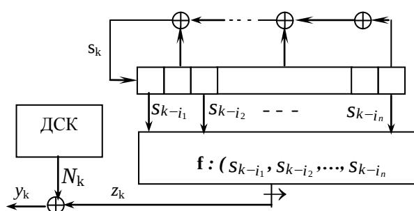
Рисунок 3 – Схема фильтр-генератора
