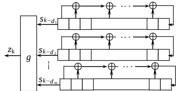
Рисунок 4 – Схема эквивалентной системы
