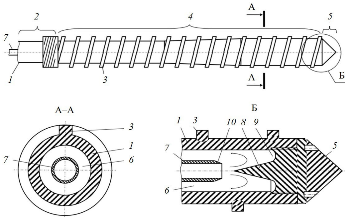
Рисунок 1 – Конструкція вузла охолодження черв'яка одночерв'ячного преса відповідно до пат. України 159256 U [16] (пояснення в тексті)
