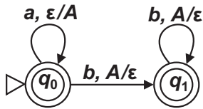
Рис. 4.11 Граф МП-автомата зображено на рис. 4.11.
