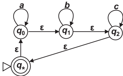
Рис. 3.33. Автомат, що допускає мову \{a^n b^m c^k : n \geq 0, m \geq 0, k \geq 0\}^*
