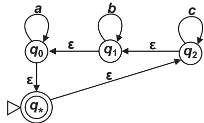
Рис. 3.34. Автомат, що допускає мову \{c^n b^m a^k : n \geq 0, m \geq 0, k \geq 0\}^*
