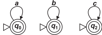
Рис. 3.32. Автомат, що допускає мову \{a^n : n \geq 0\} \cup \{b^n : n \geq 0\} \cup \{c^n : n \geq 0\}
