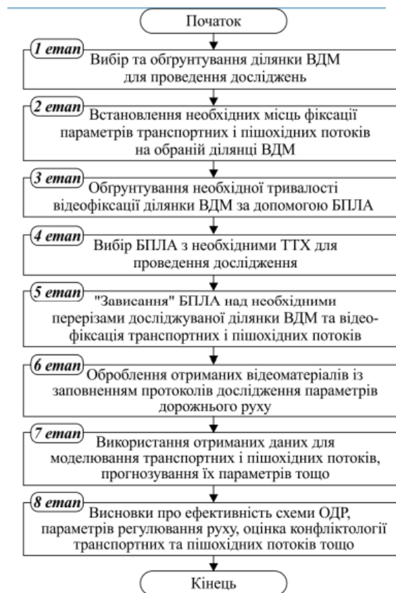
Рисунок 3.1 - Структурна схема імітаційної моделі дослідження параметрів транспортних і пішохідних потоків із використанням запропонованого способу [7]
